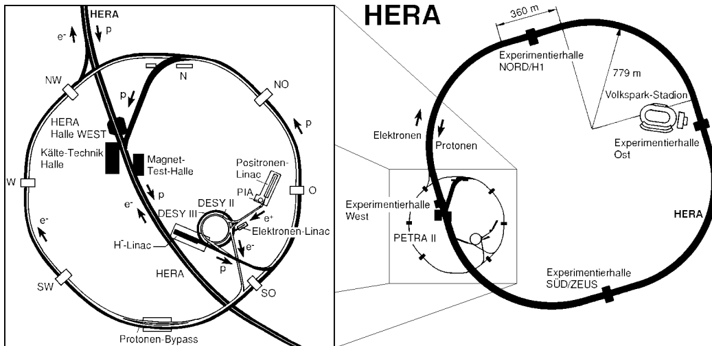
Abbildung 1.1: Die Hadron-Elektron-Ring-Anlage HERA
