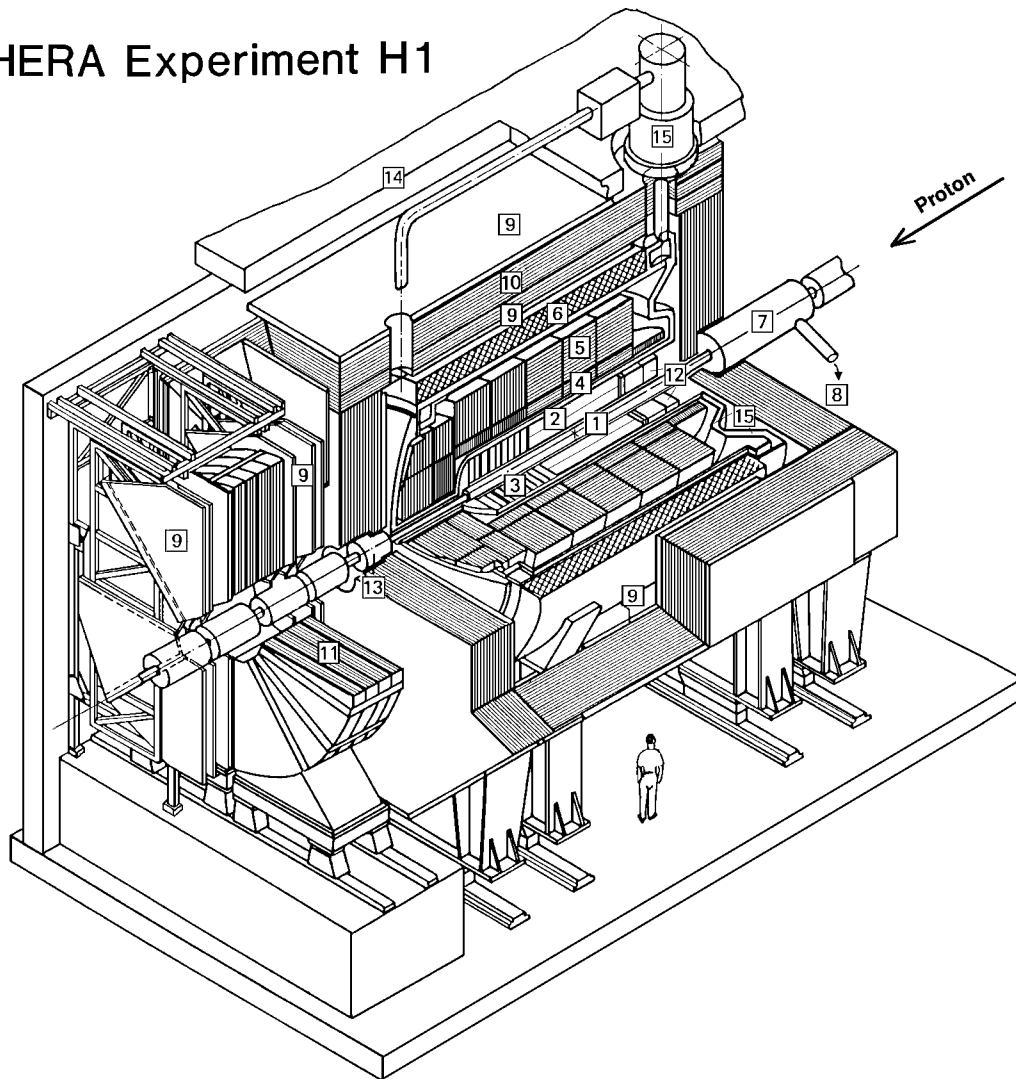
Abbildung 1.2: Der H1-Detektor
