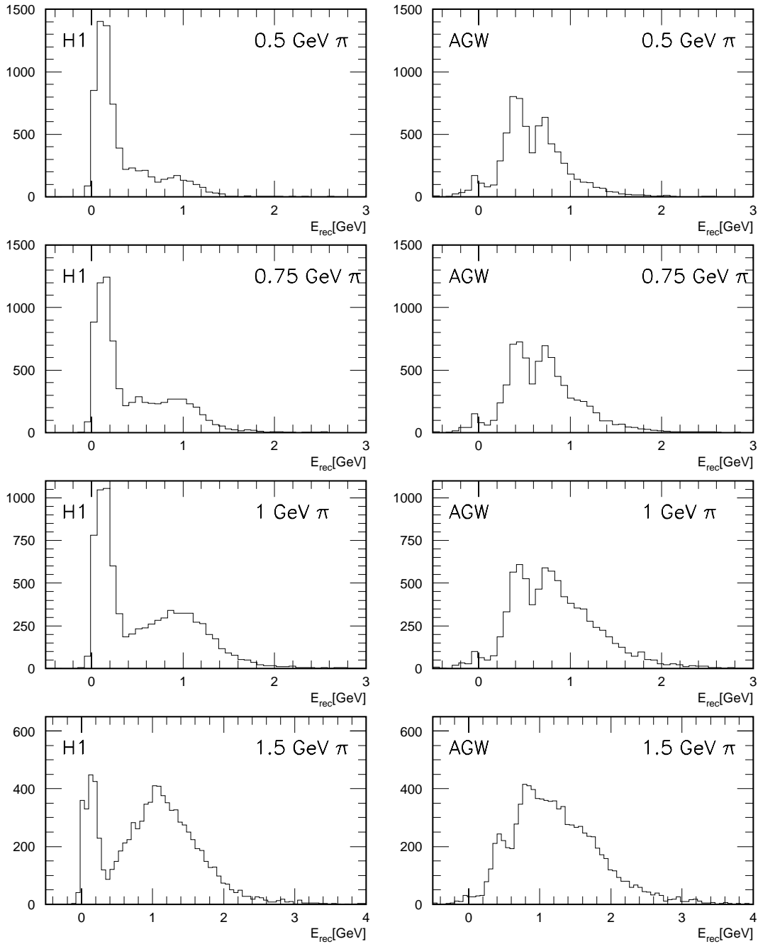
Abbildung 5.1: Verteilungen der rekonstruierten Energien für niedrige Einfallsimpulse simulierter Pionen. Die linke Spalte zeigt die Verteilungen der H1-Gewichtung (H1), die rechte Spalte die der alternativen Gewichtung (AGW).
