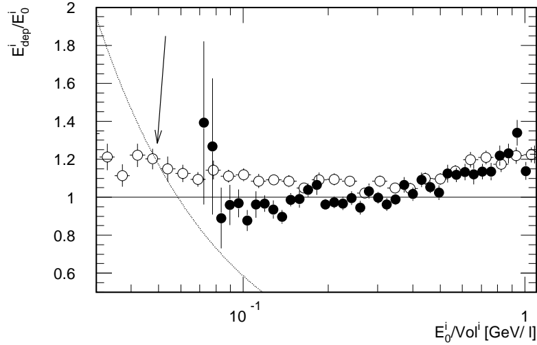
Abbildung 4.9: Erklärung des Einflusses des elektronischen Rauschens auf die Gewichtungsfaktoren bei kleinen Energiedichten. Die offenen Kreise bezeichnen Gewichtungsfaktoren ohne elektronisches Rauschen und ohne Rauschschnitt, die schwarzen Kreise entsprechen Gewichtungsfaktoren, die aus Simulationen mit elektronischem Rauschen und angewandtem Rauschschnitt berechnet worden sind. Die eingezeichnete Kurve stellt den für den ausgewählten Gewichtungsfaktor berechneten funktionalen Zusammenhang zwischen der Energiedichte und dem Gewichtungsfaktor mit E_{dep}^i = konst. dar.
