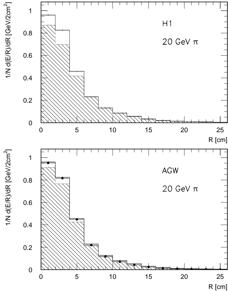
Abbildung 5.17: Radiale Energieverteilungen beider Gewichtungsverfahren für Pionen mit 20 GeV Einfallsimpuls. Die nicht schraffierte Fläche ist die insgesamt im Kalorimeter deponierte Energie. Das schraffierte Histogramm mit den gepunkteten Umrißlinien stellt die rekonstruierte Energie des jeweiligen Gewichtungsverfahrens dar. Die Verteilung, welche durch die vollen Kreise angezeigt wird, ist die Verteilung der deponierten Energien der Zellen, die nach dem Rauschschnitt verblieben sind.
