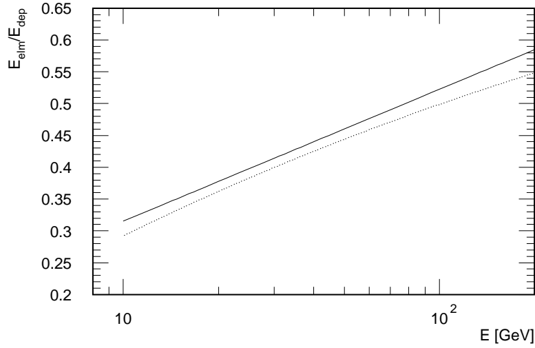
Abbildung 2.7: Der Anteil der elektromagnetisch deponierten Energie f_{elm} = E_{elm}/E_{dep} in Abhängigkeit von der Einfallsenergie E . Die durchgezogene Linie gibt die Anpassung an die simulierten Daten aus Abbildung 2.5 wieder, die gepunktete Linie zeigt den Verlauf der durch Gleichung (2.20) beschriebenen Abhängigkeit.
