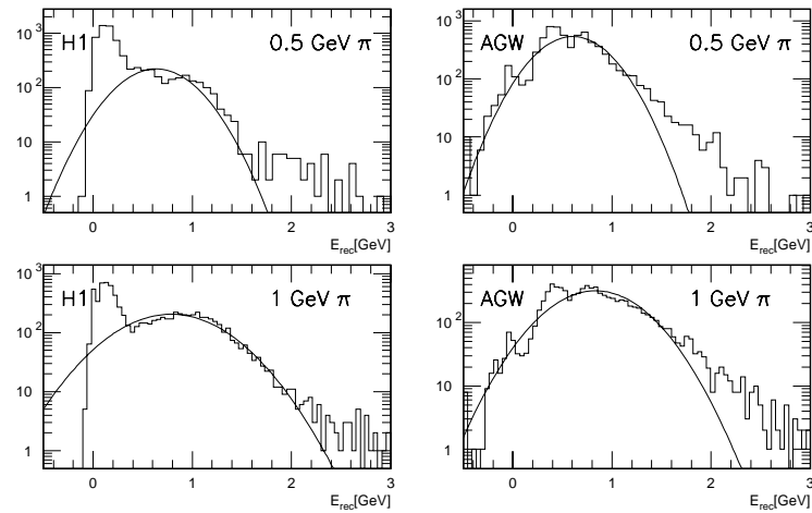
Abbildung 5.4: Verteilungen der rekonstruierten Energien für simulierte Pionen mit 0.5 GeV und 1 GeV Einfallsimpulsen in halblogarithmischer Darstellung. Die linke Spalte zeigt die Verteilungen der H1-Gewichtung (H1), die rechte Spalte die der alternativen Gewichtung (AGW). Eingezeichnet sind die an die Verteilungen angepassten Gaußfunktionen.
