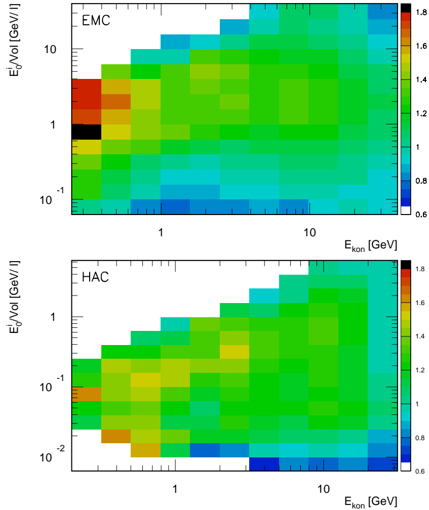
Abbildung 4.7: Ermittelte Gewichtungsfaktoren in Abhängigkeit von der Energiedichte E_0^i/Vol^i und der Kegelenergie E_{kon} für das elektromagnetische (EMC) Kalorimeter (oben) und für das hadronische (HAC) Kalorimeter (unten). Die Farbskala am rechten Rand zeigt die den Farben zugeordneten Werte der Gewichtungsfaktoren. Die weißen Flächen entsprechen Bereichen, in denen keine Gewichtungsfaktoren ermittelt werden konnten. Siehe auch Anhang A.
