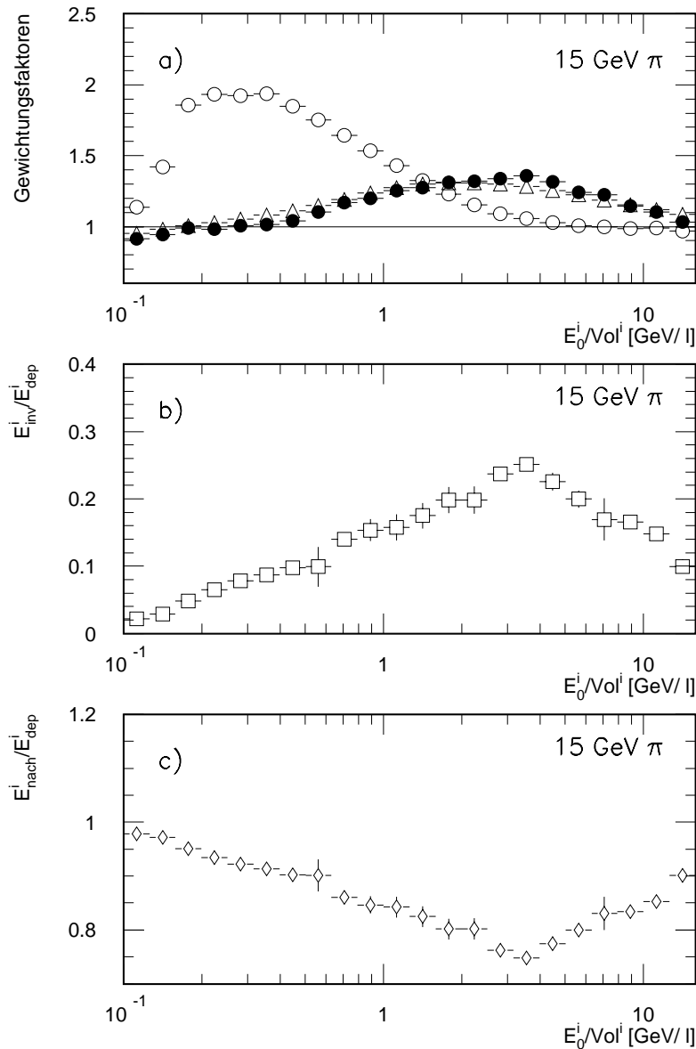
Abbildung 5.12: a) Gewichtungsfaktoren für 15 GeV-Pionen im elektromagnetischen Teil des Kalorimeters in Abhängigkeit von der Energiedichte, (○) H1-Gewichtung, (△) alternative Gewichtung, (●) ideale Gewichtungsfaktoren. b) Anteil der nicht nachweisbar deponierten Energie in den Zellen im elektromagnetischen Teil des Kalorimeters in Abhängigkeit von der Energiedichte. c) Anteil der nachweisbar deponierten Energie in den Zellen im elektromagnetischen Teil des Kalorimeters in Abhängigkeit von der Energiedichte.
