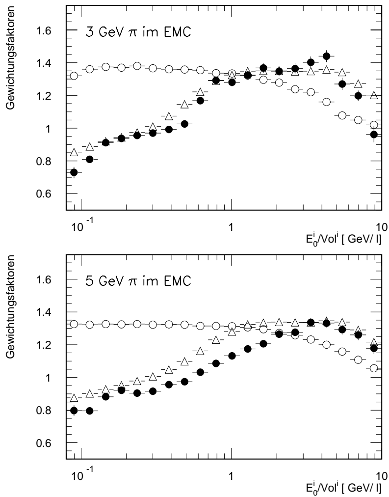
Abbildung 5.10: Vergleich der verwendeten Gewichtungsfaktoren beider Verfahren mit den idealen Gewichtungsfaktoren für 3 GeV und 5 GeV Pionen. Die Gewichtungsfaktoren der Auslesezellen im elektromagnetischen Teil (EMC) des Kalorimeters sind in Abhängigkeit von der Energiedichte zu sehen:
