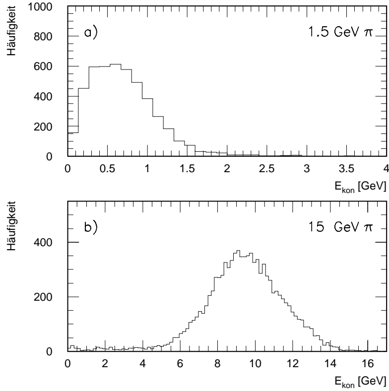
Abbildung 4.4: Verteilung der Energien der energiereichsten Kegel für 1.5 GeV (a) und 15 GeV (b) Pionen.
