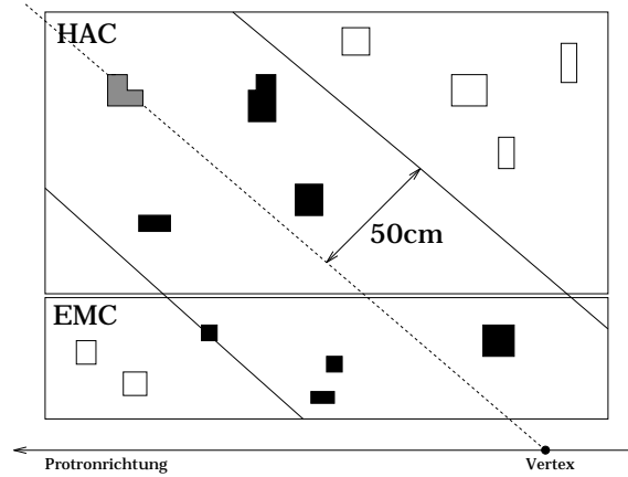
Abbildung 3.5: Zusammenfassung hadronischer Cluster zu hadronischen Objekten. Das schraffierte Vieleck sei der energiereichste hadronische Cluster. Die schwarzen Vielecke stellen hadronische Cluster dar, die zu dem hadronischen Objekt des energiereichsten Clusters gehören.
