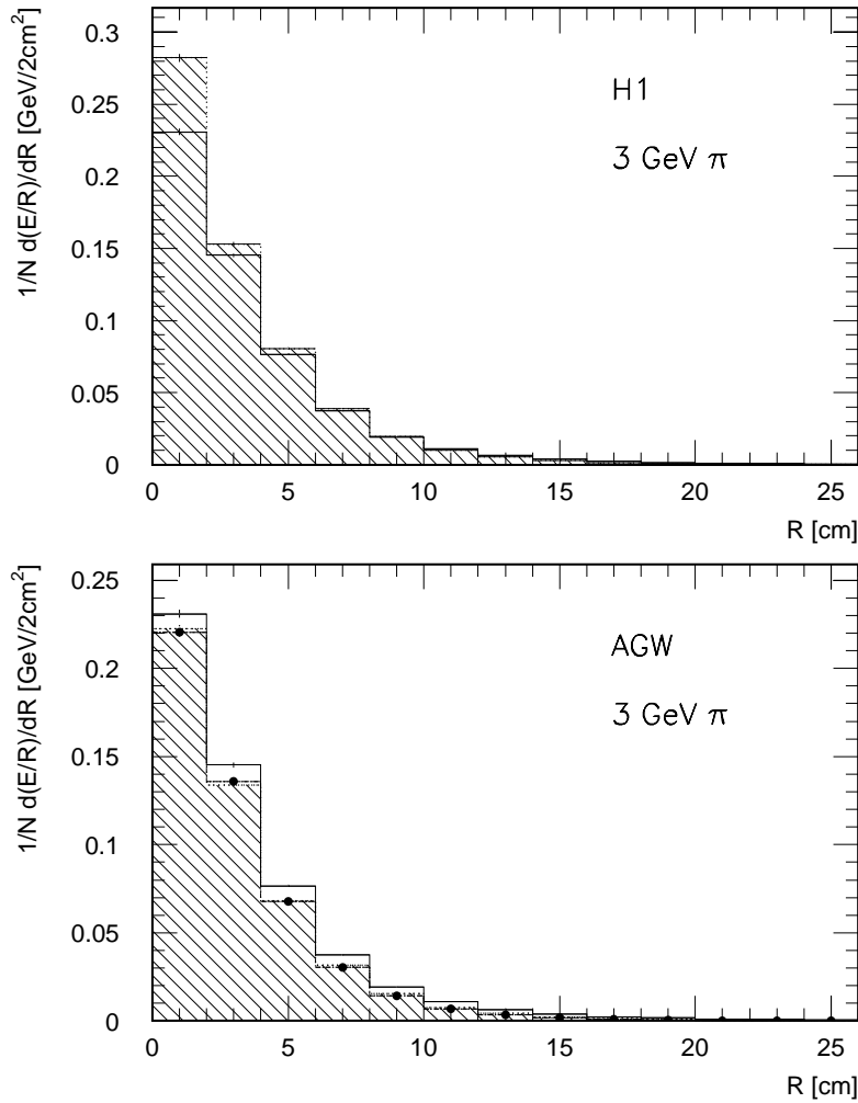
Abbildung 5.16: Radiale Energieverteilungen beider Gewichtungungsverfahren für Pionen mit 3 GeV Einfallsimpuls. Die nicht schraffierte Fläche stellt die insgesamt im Kalorimeter deponierte Energie dar. Das schraffierte Histogramm mit den gepunkteten Umrißlinien zeigt die rekonstruierte Energie des jeweiligen Gewichtungungsverfahrens. Die Verteilung der deponierten Energie der Zellen, die nach der Rauschunterdrückung verblieben sind, wird durch volle Kreise repräsentiert.
