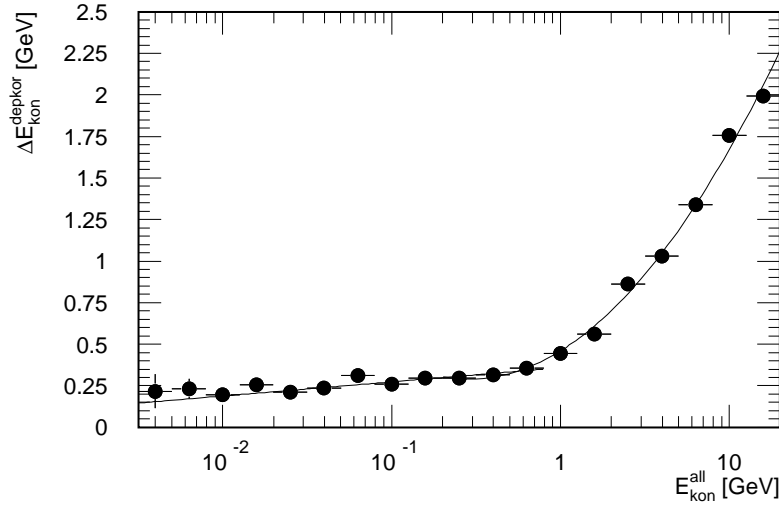
Abbildung 4.10: Mittlerer Energieverlust \Delta E_{kon}^{depkor} in Abhängigkeit von der Kegelenergie E_{kon}^{all} . Die eingezeichnete Kurve zeigt die angepaßten Parametrisierungen.
