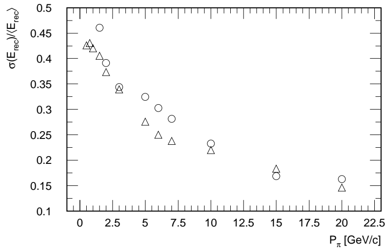
Abbildung 5.8: Relative Auflösung der rekonstruierten Energien beider Verfahren. (o) H1-Gewichtung, ( \Delta ) alternative Gewichtung.
