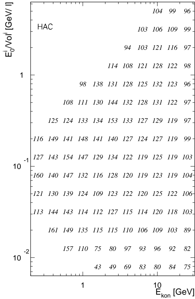
Abbildung A.2: Werte der Gewichtungsfaktoren (vergleiche Abbildung 4.7) in Prozent für das hadronische (HAC) Kalorimeter in Abhängigkeit von der Energiedichte E_0^i/Vol^i und der Kegelernergie E_{kon} .
