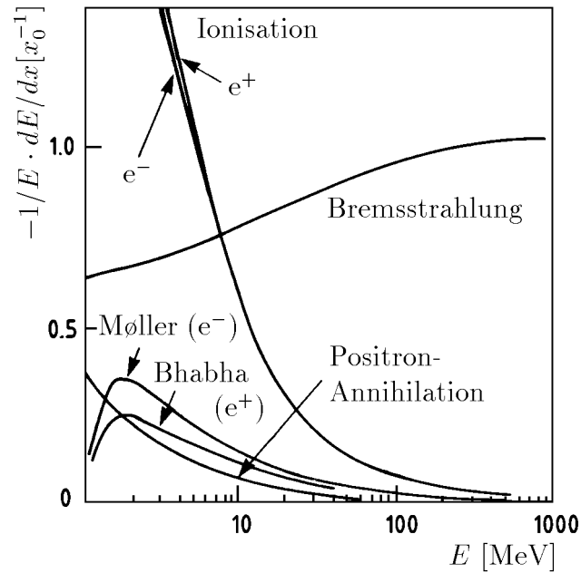
Abbildung 2.1: Energieverlustmechanismen für Elektronen, bzw. Positronen in Blei in Abhängigkeit von der Elektronen-/Positronenenergie [Par 90]. (Møller-Streuung: e^-e^- \rightarrow e^-e^- ; Bhabha-Streuung: e^+e^- \rightarrow e^+e^- ; Positronen-Annihilation: e^+e^- \rightarrow \gamma\gamma )
