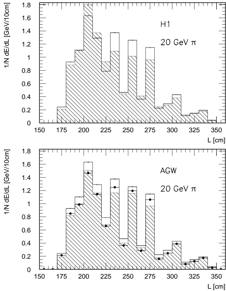
Abbildung 5.15: Longitudinale Energieverteilungen beider Gewichtungungsverfahren für Pionen mit 20 GeV Einfallsimpuls. Die nicht schraffierte Fläche ist die im Kalorimeter deponierte Energie. Die schraffierte Fläche mit gepunkteten Umrislinien ist die rekonstruierte Energie des jeweiligen Gewichtungungsverfahrens. Die Verteilung, welche durch die vollen Kreise angezeigt wird, ist die Verteilung der deponierten Energien der Zellen, die nach dem Rauschschnitt verblieben sind.
