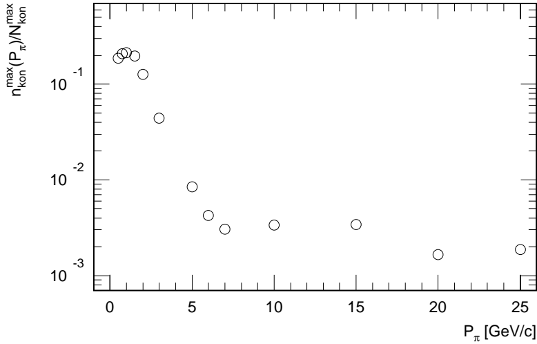
Abbildung 4.5: Verhältnisse der energiereichsten Kegel der jeweiligen Pionimpulse zur Gesamtzahl der in das Intervall E_{kon} \in [0, 1] \text{ GeV} eingetragenen energiereichsten Kegel als Funktion aller simulierten Pionimpulse.
