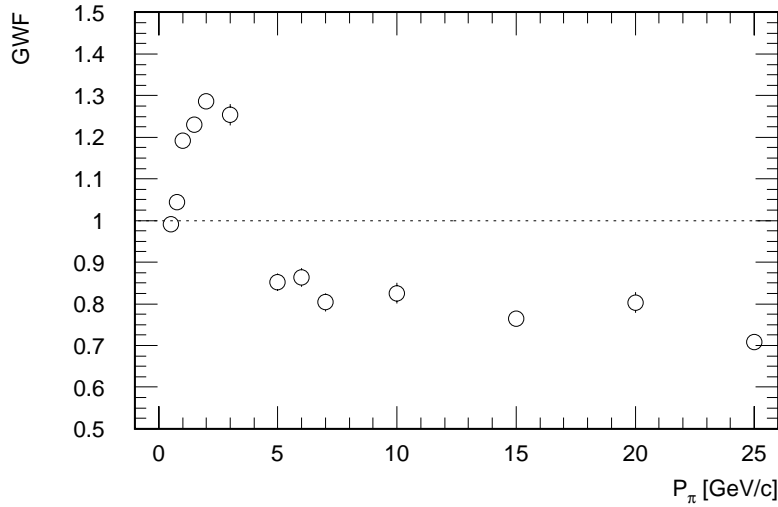
Abbildung 4.2: Gewichtungsfaktor GWF für E_{kon} \in [0, 1] \text{ GeV} und \rho^i \in [0, 1] \text{ GeV/l} in Abhängigkeit vom Einfallsimpuls des Pions.
