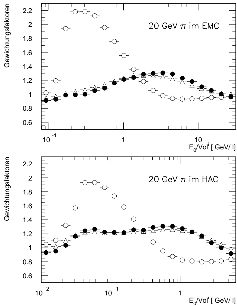
Abbildung 5.11: Vergleich der verwendeten Gewichtungsfaktoren beider Verfahren mit den idealen Gewichtungsfaktoren für 20 GeV Pionen im elektromagnetischen (EMC) und hadronischen (HAC) Teil des Kalorimeters in Abhängigkeit von der Energiedichte der Auslesezellen:
