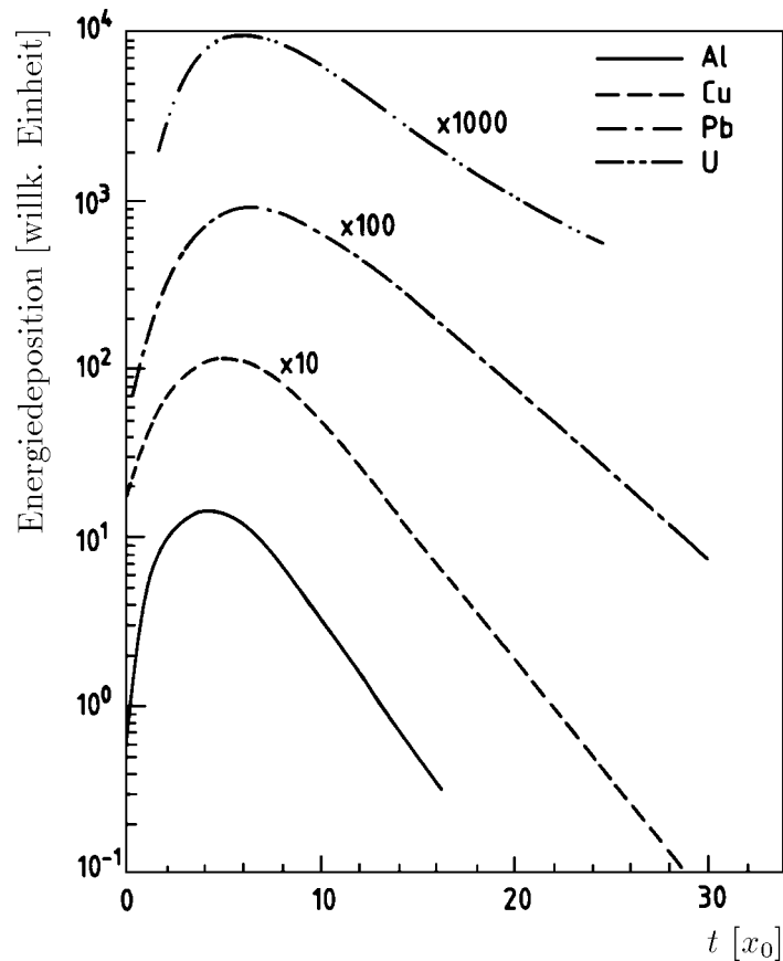
Abbildung 2.3: Longitudinales Schauerprofil für 6 GeV Elektronen in Aluminium, Blei, Kupfer und Uran [Fab 85b].
