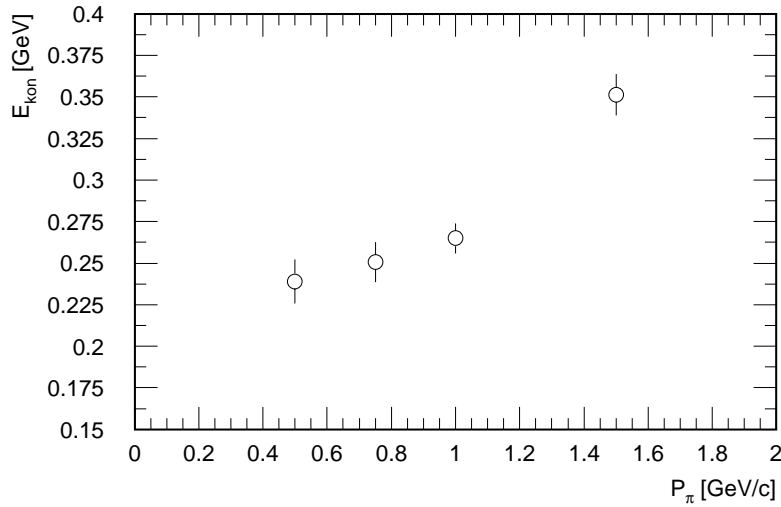
Abbildung 4.11: Mittlere Kegelergie für Ereignisse, in denen weniger als 40% der Einfallenergie im Kalorimeter deponiert worden ist. Zu sehen sind die Mittelwerte für Pionen mit Einfallsimpulsen von 0.5 GeV, 0.75 GeV, 1.0 GeV und 1.5 GeV.
