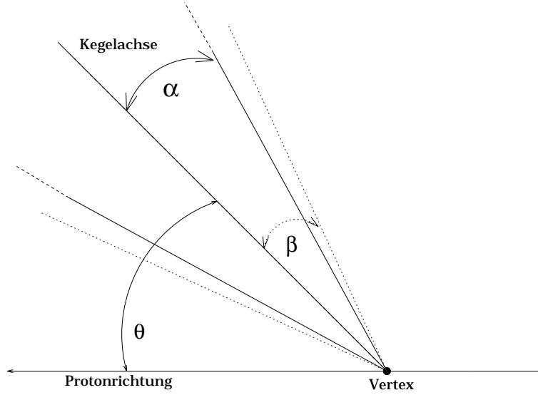
Abbildung 3.7: \alpha - und \beta -Kegel der iterativen Gewichtung.
