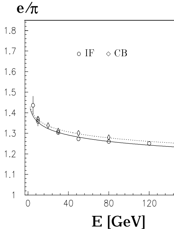
Abbildung 3.4: Mit Hilfe von Simulationen berechnete e/\pi Verhältnis des H1-Kalorimeters für die IF- und CB-Module in Abhängigkeit von der Einschussenergie [LAR 93b].
