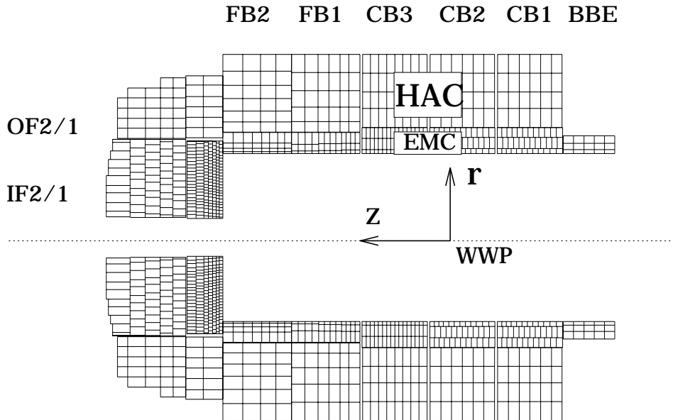
Abbildung 3.3: Auslesezellen im elektromagnetischen (EMC) und hadronischen (HAC) Teil des H1-Kalorimeters in longitudinaler und radialer Richtung
