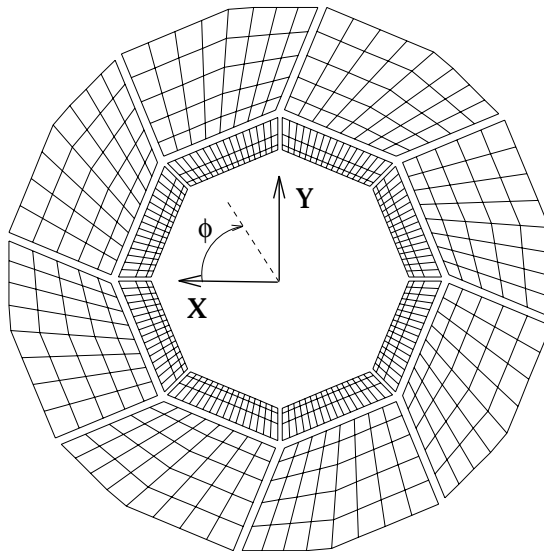
Abbildung 3.2: Segmentierung des H1-Kalorimeters im elektromagnetischen (innere Module) und im hadronischen (äußere Module) Teil des H1-Kalorimeters in der r - \phi -Ebene
