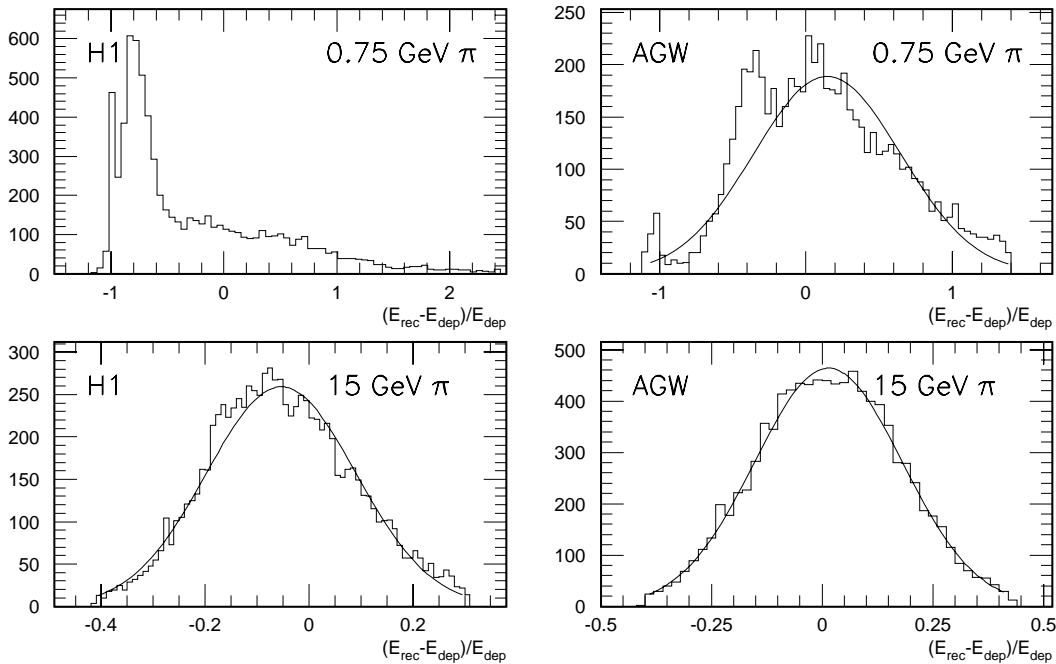
Abbildung 5.7: Verteilungen der Größe (E_{rec} - E_{dep})/E_{dep} des H1-Gewichtungsverfahrens und der alternativen Gewichtung für Pionen mit Einfallsimpulsen von 0.75 GeV und 15 GeV.
