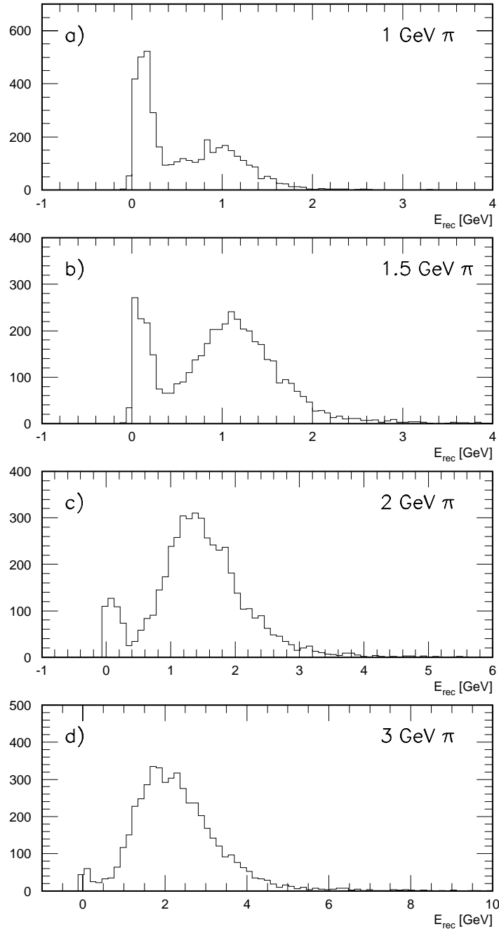
Abbildung 3.10: Verteilungen der rekonstruierten Energie mit der H1-Gewichtung für simulierte Pionen mit verschiedenen Impulsen 1 GeV, 1.5 GeV, 2 GeV und 3 GeV.
