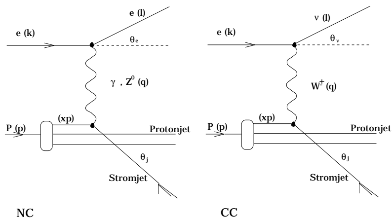
Abbildung 1.3: Neutraler Strom (NC) und geladener Strom (CC) in der tiefinelastischen Elektron-Proton-Streuung. Die Viererimpulse der Teilchen sind in Klammern angegeben.
