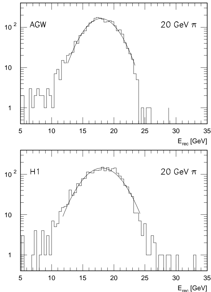
Abbildung 5.13: Am CERN-Teststrahl gemessene Energieverteilung der Pionen mit 20 GeV Einfallsimpulsen in halblogarithmischer Darstellung. Die obere Abbildung zeigt die mit der alternativen Gewichtung (AGW) rekonstruierten Energien. Die untere Abbildung zeigt die mit der H1-Gewichtung rekonstruierten Energien. An beide Verteilungen wurden Gaußfunktionen angepaßt.
