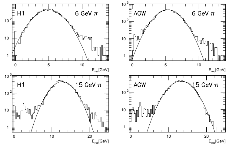
Abbildung 5.5: Verteilungen der rekonstruierten Energien für simulierte Pionen mit 6 GeV und 15 GeV Einfallsimpulsen in halblogarithmischer Darstellung. Links: Verteilungen H1-Gewichtung (H1) Rechts: Verteilungen der alternativen Gewichtung (AGW) Eingezeichnet sind die an die Verteilungen angepassten Gaußfunktionen.
