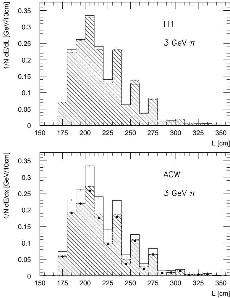
Abbildung 5.14: Longitudinale Energieverteilungen beider Gewichtungungsverfahren für Pionen mit 3 GeV Einfallsimpuls. Das nicht schraffierte Histogramm zeigt die im Kalorimeter deponierte Energie. Die schraffierte Fläche mit gepunkteten Umrißlinien stellt die rekonstruierte Energie des jeweiligen Gewichtungungsverfahrens dar. Die Verteilung der deponierten Energie in Zellen, die nach der Rauschunterdrückung verblieben sind, wird durch volle Kreise repräsentiert.
