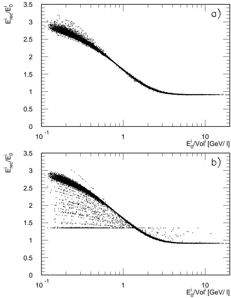
Abbildung 3.9: Verwendete Gewichtungsfaktoren E_{rec}^i/E_0^i in Abhängigkeit von der Energiedichte für simulierte 20GeV-Pionen. Die obere Abbildung a) zeigt die Gewichtungsfaktoren des iterativen Gewichtungsansatzes. Die untere Abbildung b) zeigt die Gewichtungsfaktoren aus der Kombination beider Gewichtungsansätze.
