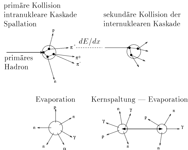
Abbildung 2.4: Entwicklung eines hadronischen Schauers nach dem Spallationsmodell [Zei 91].
