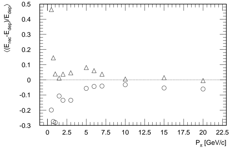
Abbildung 5.6: Linearitäten L beider Verfahren als Funktion des Einfallsimpulses der Pionen, (o) H1-Gewichtung, ( \Delta ) alternative Gewichtung. Die statistischen Fehler sind kleiner als die Symbolgrößen.
