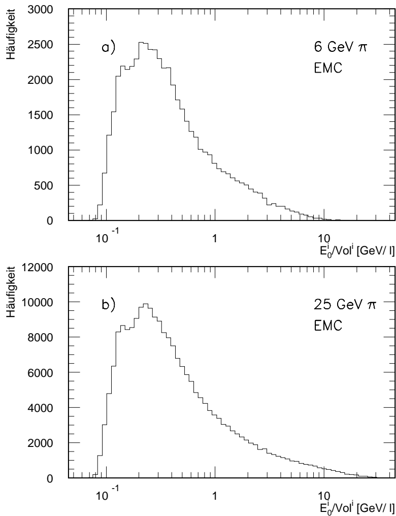
Abbildung 4.6: Verteilung der Energiedichten in den Zellen der energiereichsten Kegel für 6 GeV Pionen in a) und 25 GeV Pionen b) als Funktion von E_0^i/Vol^i mit logarithmischer Abszisse.
