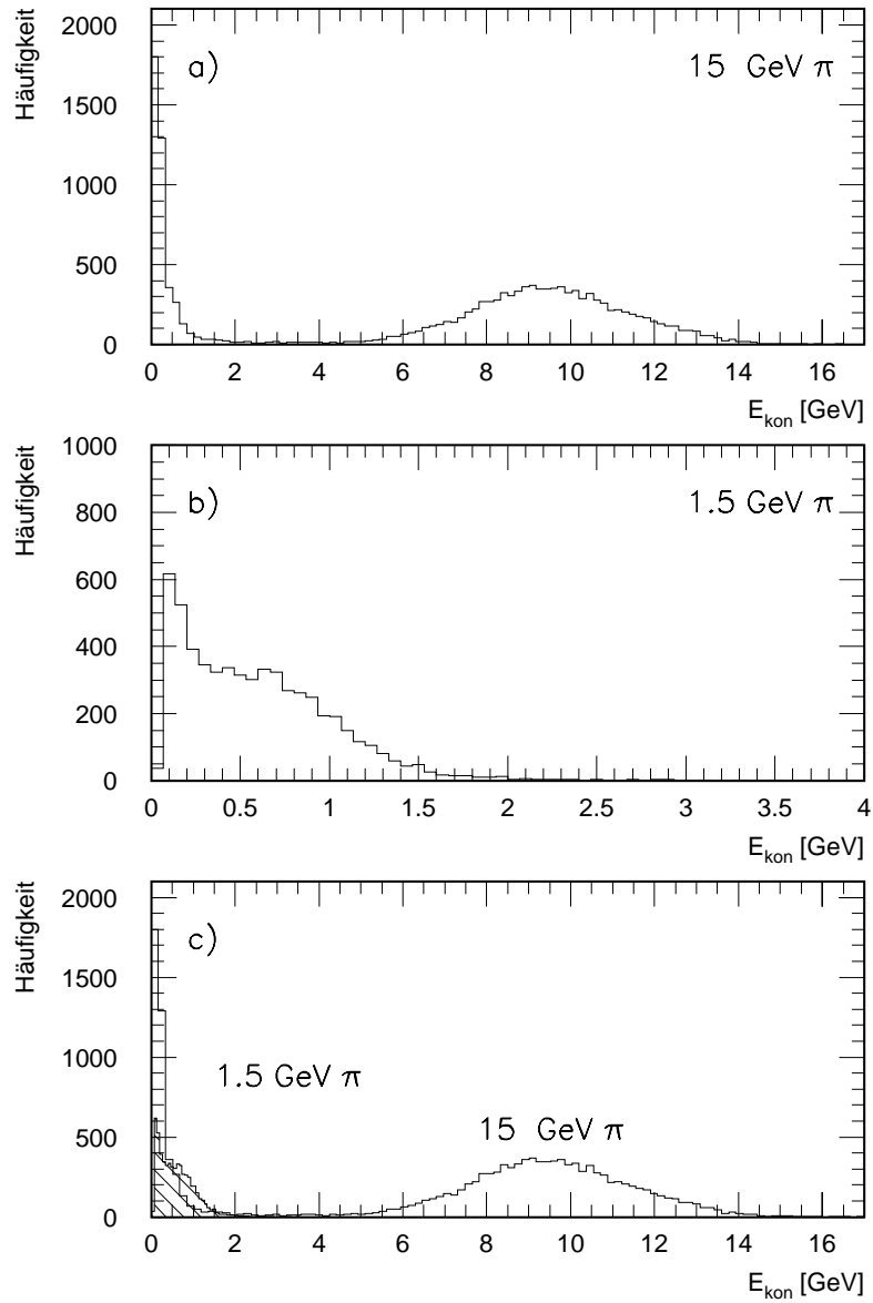
Abbildung 4.1: Verteilungen der Kegelergien auf elektromagnetischer Skala für Pionen mit a) 15 GeV und b) 1.5 GeV Einfallsimpulsen, sowie die Überlagerung beider Verteilungen c).
