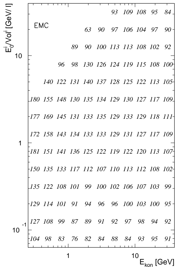
Abbildung A.1: Werte der Gewichtungsfaktoren (vergleiche Abbildung 4.7) in Prozent für das elektromagnetische (EMC) Kalorimeter in Abhängigkeit von der Energiedichte E_0^i/Vol^i und der Kegelenergie E_{kon} .
