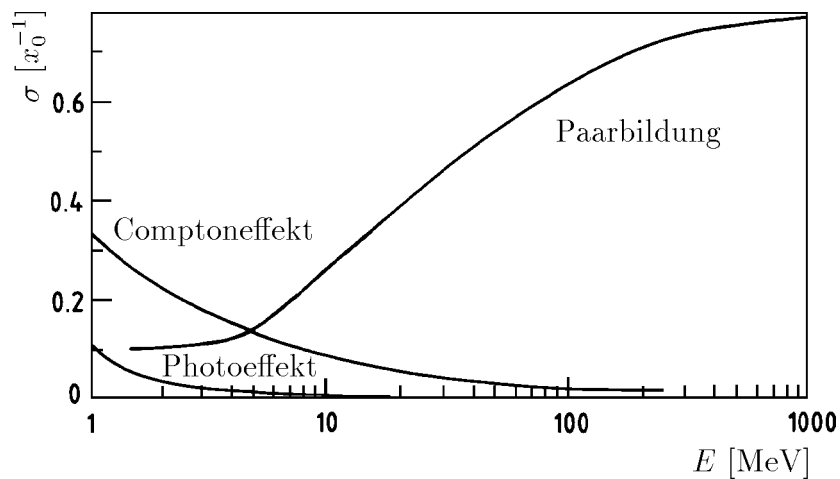
Abbildung 2.2: Wechselwirkungswahrscheinlichkeiten auf einer Strahlungslänge der Photoabsorption in Blei [Par 90].
