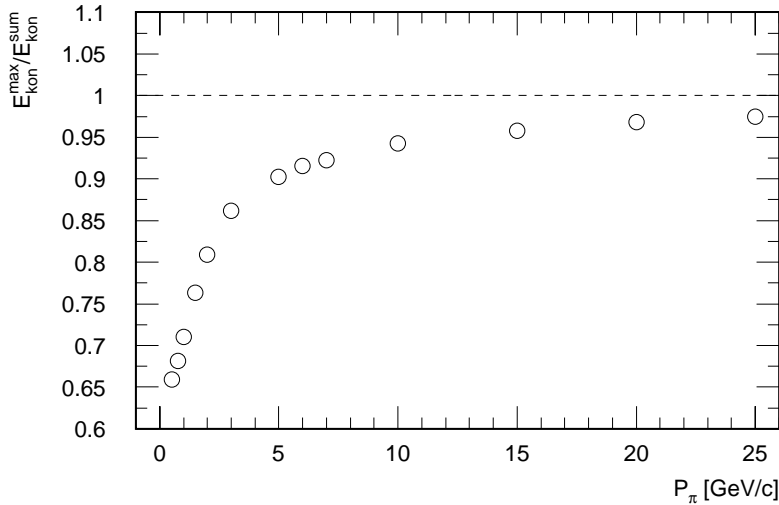
Abbildung 4.3: Anteil der Energie des energiereichsten Kegels E_{kon}^{max} an der insgesamt von allen Kegeln des Ereignisses getragenen Energie E_{kon}^{sum} für Ereignisse mit mehr als einem Kegel. Die Anteile sind in Abhängigkeit vom Einfallsimpuls des Pions aufgetragen. Die statistischen Fehler sind kleiner als die Symbolgröße.
