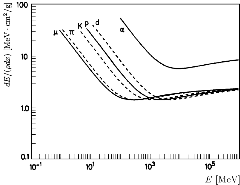
Abbildung 2.8: Ionisationsverlust schwerer Teilchen in Abhängigkeit von der Energie [Leo 87].
