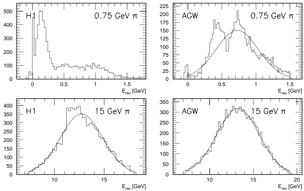
Abbildung 5.9: Verteilungen der rekonstruierten Energien beider Gewichtsverfahren für 0.75 GeV und 15 GeV Pionen.
