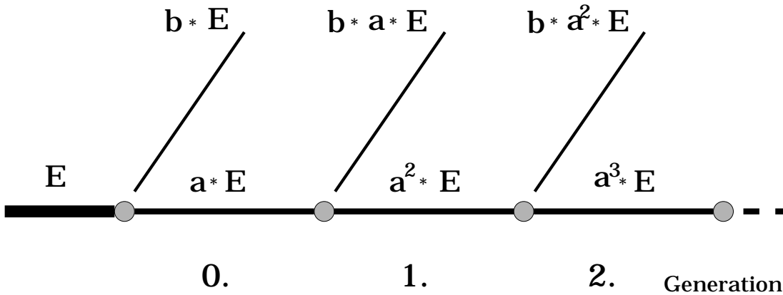
Abbildung 2.6: Energiefluß in einem einfachen Modell für hadronische Schauer.
