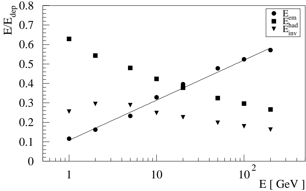
Abbildung 2.5: Anteile der drei Energiekomponenten an der deponierten Energie in hadronischen Schauern von Protonen in Abhängigkeit von der Primärenergie E . Die Protonereignisse wurden mit CALOR in einem Stahlblock simuliert [Spi 94].
