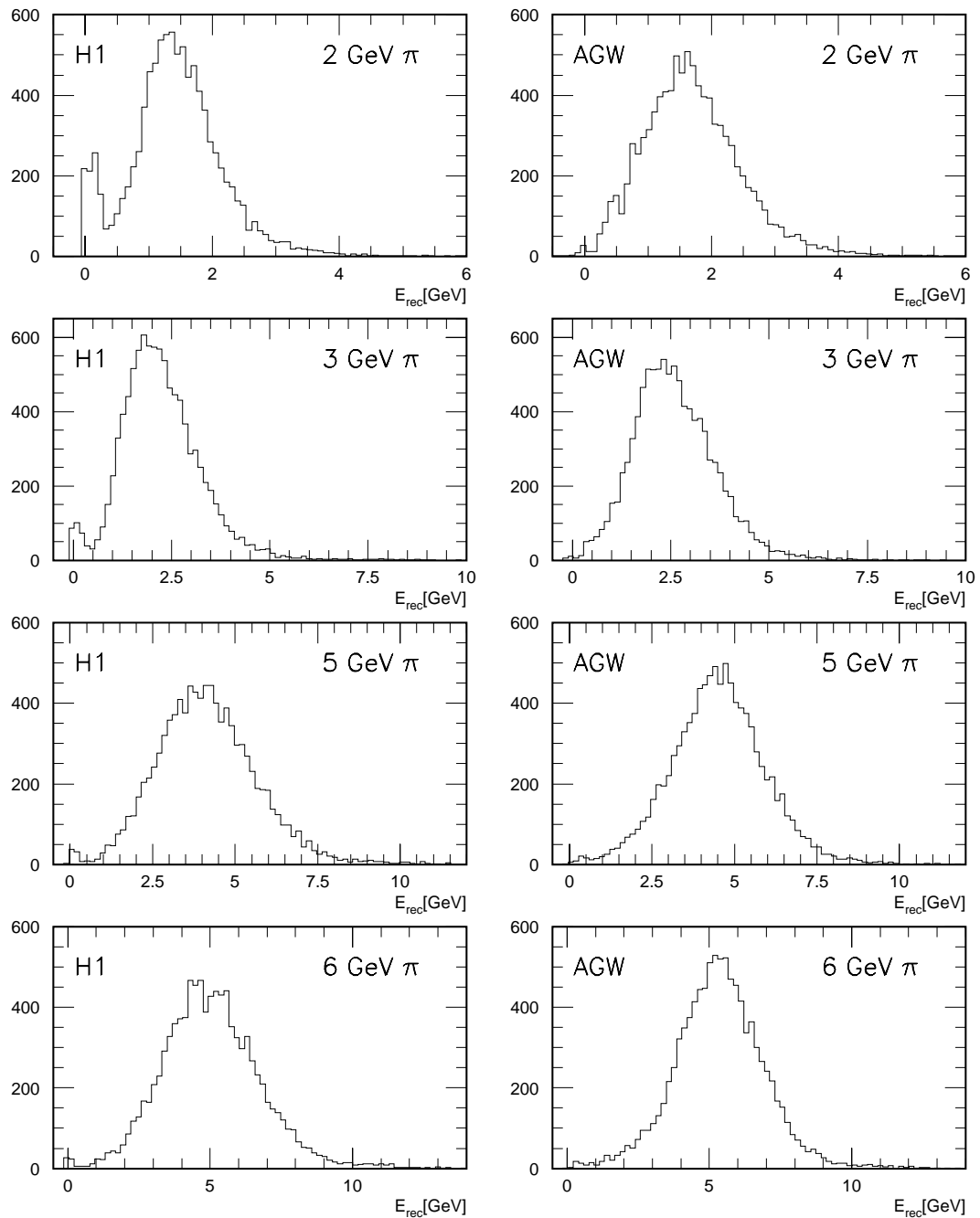
Abbildung 5.2: Verteilungen der rekonstruierten Energien für Einfallsimpulse zwischen 2 und 6 GeV für simulierte Pionen. Links sind die Verteilungen der H1-Gewichtung (H1) zu sehen, rechts daneben befinden sich die Verteilungen der alternativen Gewichtung (AGW).
