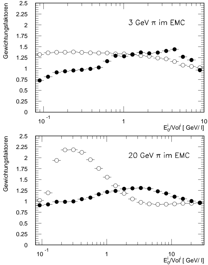
Abbildung 3.11: Vergleich der H1-Gewichtungsfaktoren E_{rec}^i/E_0^i ( \circ ) mit den idealen Gewichtungsfaktoren E_{dep}^i/E_0^i ( \bullet ) im elektromagnetischen Teil des FB-Kalorimeters für simulierte Pionen mit 3 GeV und 20 GeV Impulsen.
