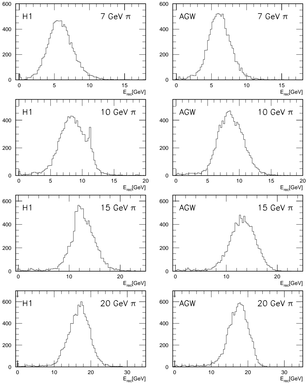
Abbildung 5.3: Verteilungen der rekonstruierten Energien für große Einfallsimpulse simulierter Pionen. Die linke Spalte zeigt die Verteilungen der H1-Gewichtung (H1), die rechte Spalte die der alternativen Gewichtung (AGW).
