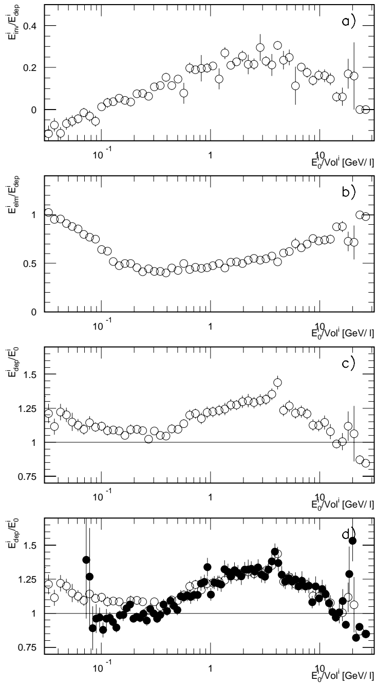
Abbildung 4.8: Vergleich der Simulation mit elektronischen Rauschen und Rauschschnitt ( \bullet ) mit der reinen Simulation ( \circ ). Erläuterungen erfolgen im Text.
