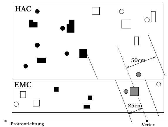
Abbildung 3.6: Beispiel für die Zuordnung der Zellen. Zellen (Kreise), die sich nicht in elektromagnetischen oder hadronischen Clustern befinden, werden, falls sie in der Nähe eines hadronischen Clusters sind, dem hadronischen Objekt (Gruppe aus dunklen Vielecken und Kreisen) dieses hadronischen Clusters zugeordnet. Die schraffierten Kreise bezeichnen Zellen, die in Bearbeitung sind.
