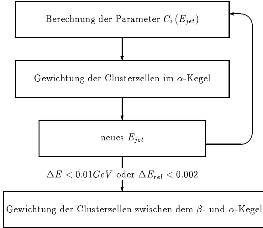
Abbildung 3.8: Flußdiagramm der iterativen Gewichtung
