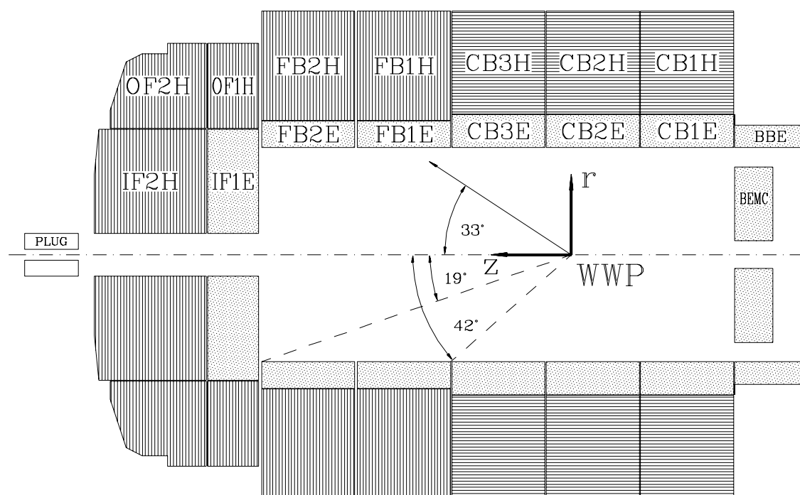
Abbildung 3.1: Schnitt durch das H1-Kalorimeter parallel zur Strahlachse.
