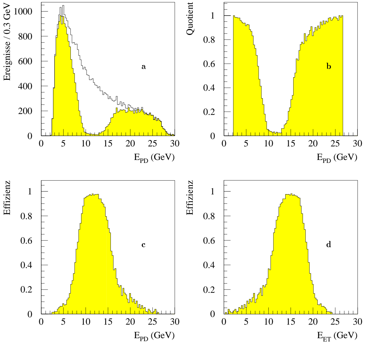
Abb. 3.10: Effizienz des Luminositäts-Systems
