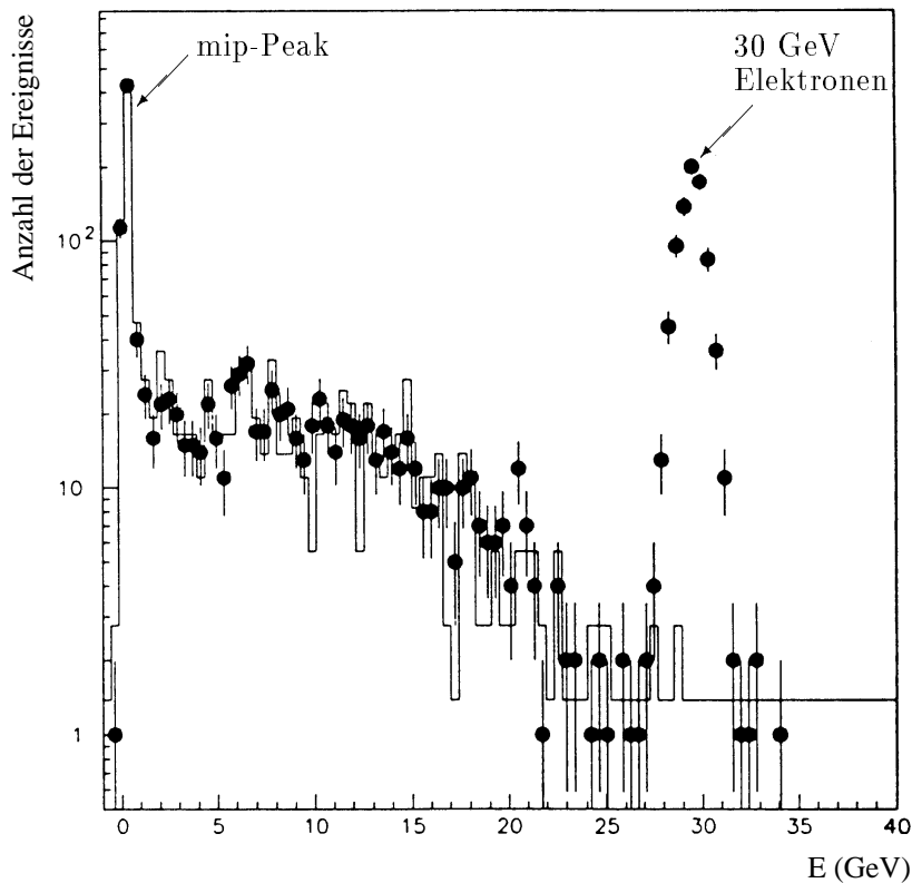
Abb. 3.14: Energiedeposition von 30 GeV-Pionen in einem BEMC Modul
