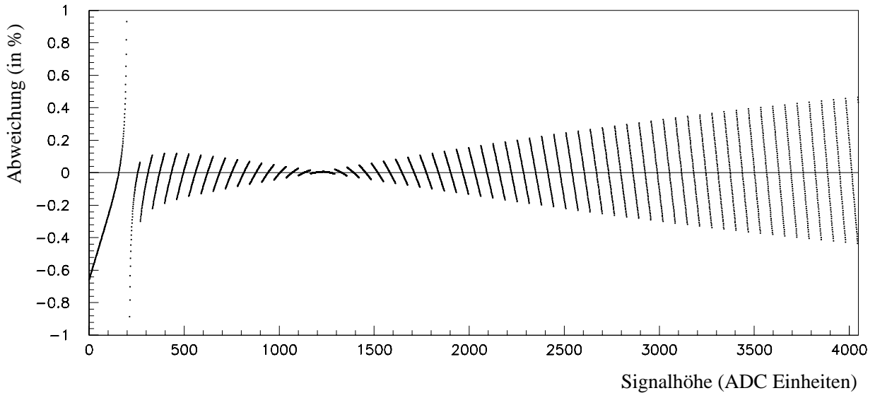
Abb. A.13: Abweichungen aufgrund der Korrekturrechnungen im DSP Für Stack 61 Diode 3 sind die Abweichungen der näherungsweise Berechnung von den exakt berechneten Werten für alle ADC-Werte in % angegeben. [Pic92]
