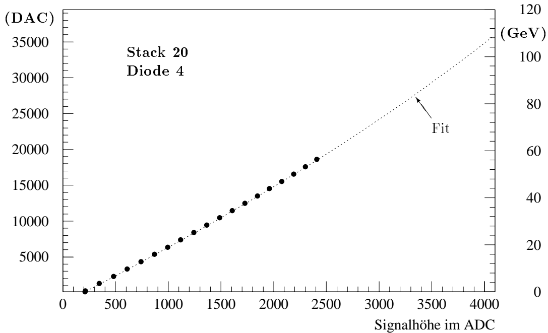
Abb. A.6: Kalibration eines elektronischen Kanals des BEMC
