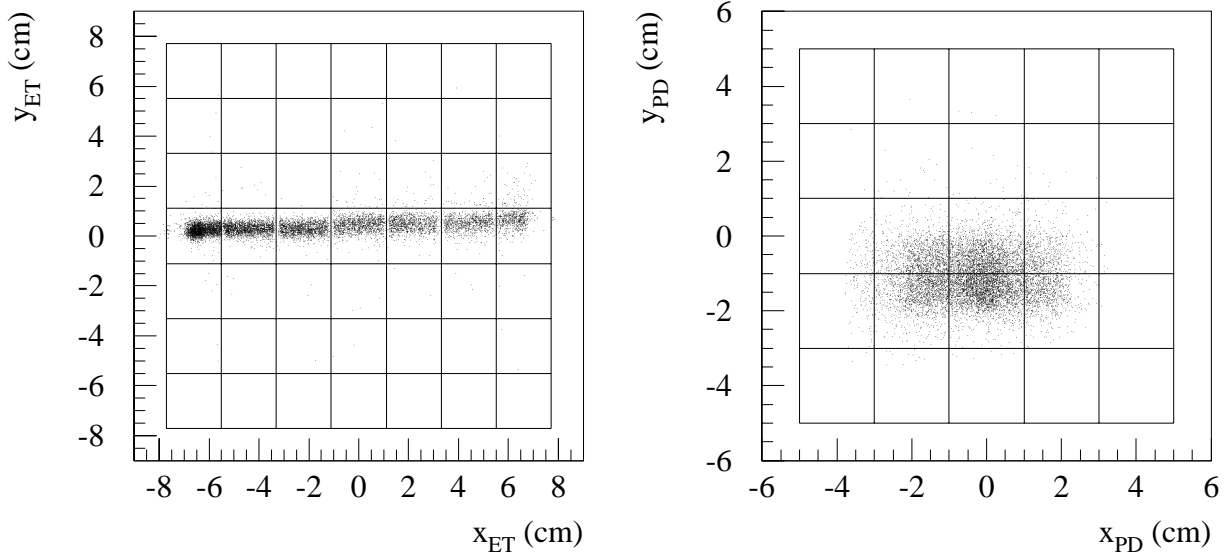
Abb. 3.8: Rekonstruierte Clusterschwerpunkte im ET und im PD
