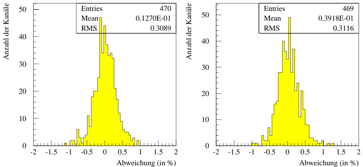
Abb. A.8: Stabilität der Pedestals
