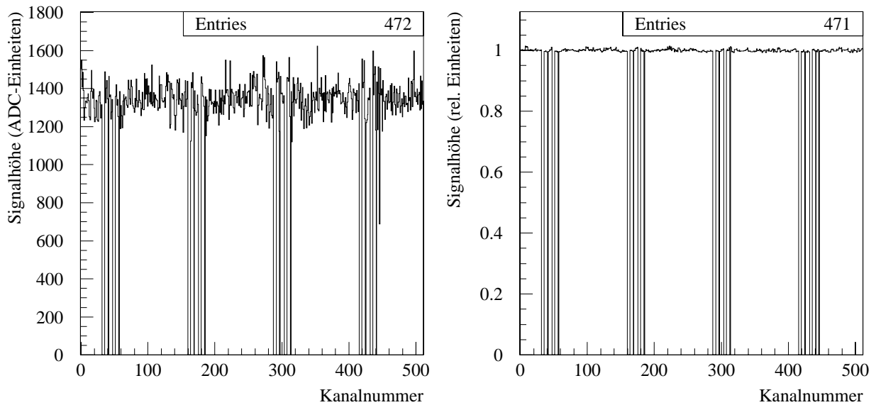
Abb. A.15: Signale der Dioden vor und nach der Korrektur im DSP
