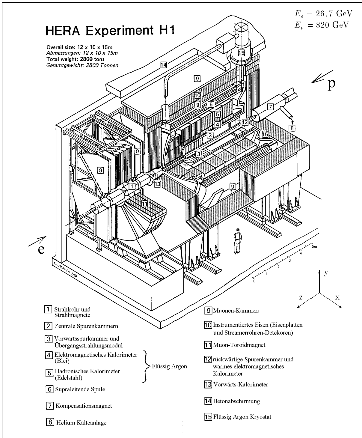
Abb. 3.2: Der H1-Detektor Perspektivische Darstellung aus [H1C86]
