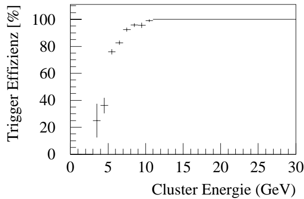
Abb. 3.16: Triggereffizienz für den energiereichsten Cluster im BEMC Die Effizienz wurde in [Kur93] für tief inelastische Ereignisse mit einem Q^2 < 100 \text{ GeV}^2 bestimmt.
