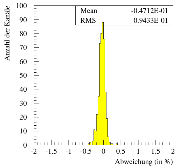
Abb. A.11: Stabilität der Energiemessung bei ca. 30 GeV Alle funktionsfähigen Kanäle zeigen eine Stabilität von besser als 1 Promille über den betrachteten Zeitraum von 2 Monaten.
