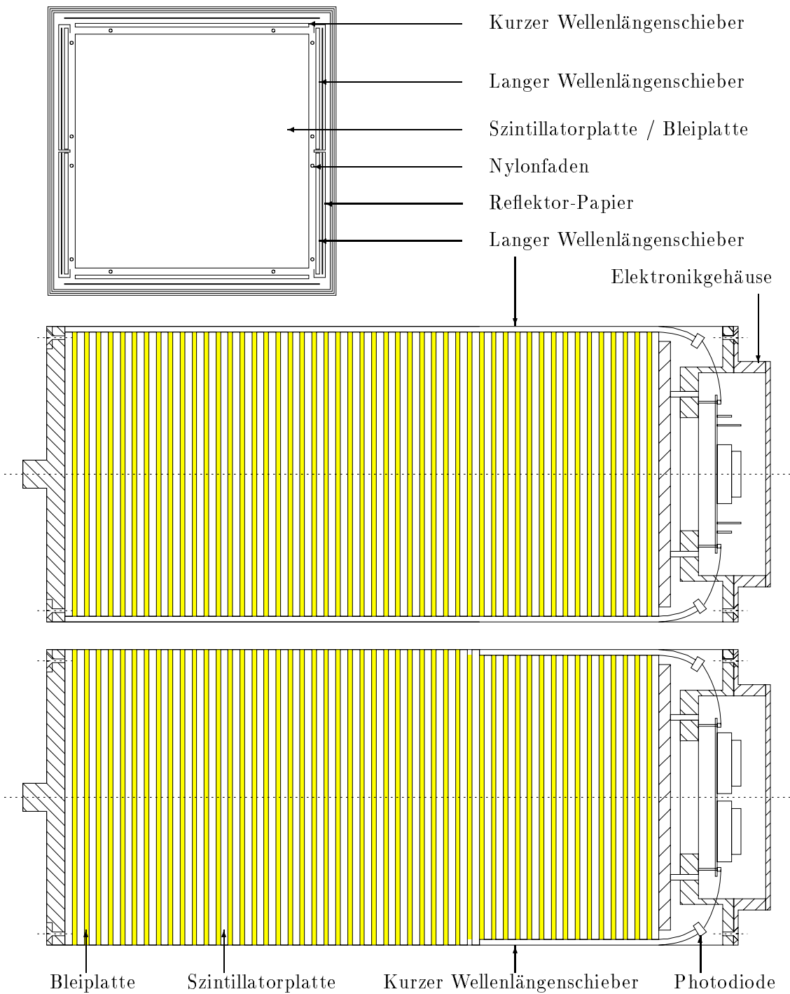
Abb. 3.13: Schnitt durch ein BEMC-Modul mit quadratischem Querschnitt
