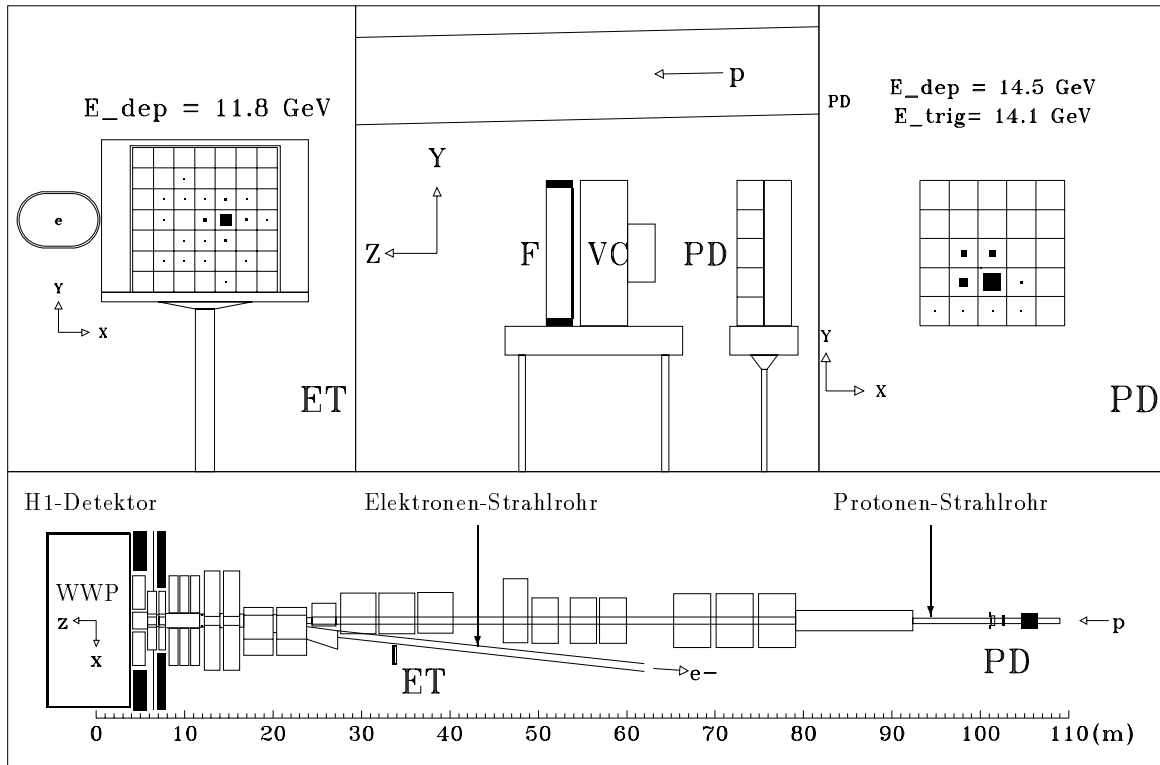
Abb. 3.4: Bremsstrahlungsreaktion im Luminositäts-System
