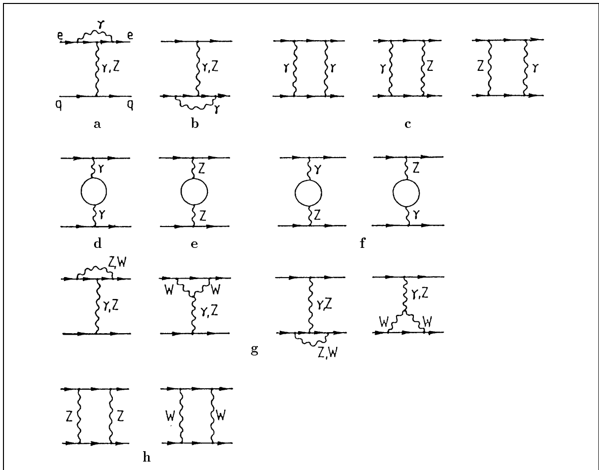
Abb. 2.3: Diagramme von Strahlungskorrekturen der Ordnung O(\alpha)
