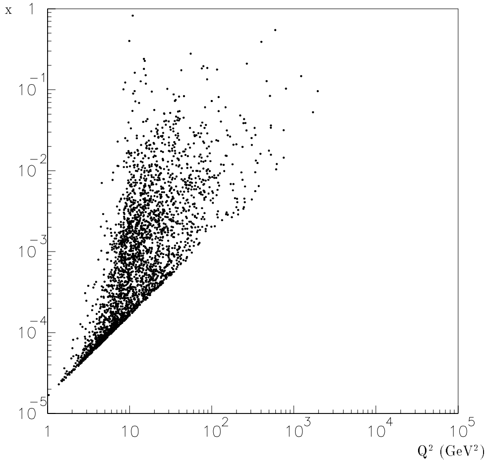
Abb. 1.2: Verteilung von Ereignis-Kandidaten in der kinematischen Ebene Die eingezeichneten Punkte zeigen für die im Herbst 1992 aufgezeichneten Ereignisse die Lage in der kinematischen Ebene. Die eingetragenen Ereignisse wurden mit der Forderung selektiert, daß eine Energie von mindestens 8 GeV in einem Kalorimeter deponiert wurde und diese Energiedeposition als gestreutes Elektron identifiziert wurde. Bei kleinem x und kleinem Q^2 ist der Wirkungsquerschnitt besonders groß. [DeR93]
