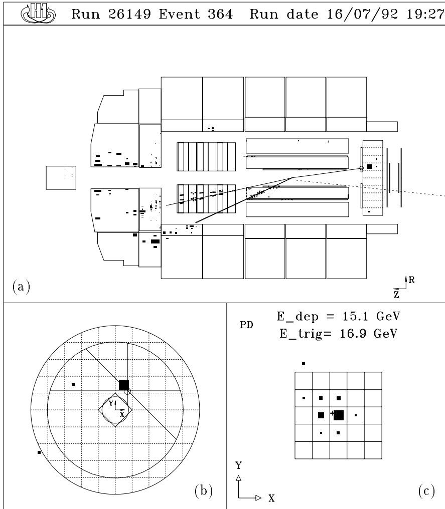
Abb. 4.1: Tief inelastisches Ereignis mit Abstrahlung eines Photons kollinear zum einlaufenden Elektron bei kleinem Q^2
