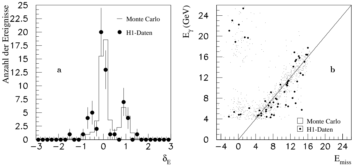
Abb. 4.5: Verteilungen bei Untergrundunterdrückung mit Hilfe des ETs
