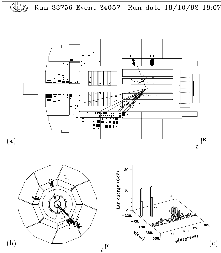
Abb. 4.14: Radiatives, tief inelastisches Ereignis mit hohem Q^2 Zur Kinematik dieses Ereignisses siehe Tab. 4.1.
