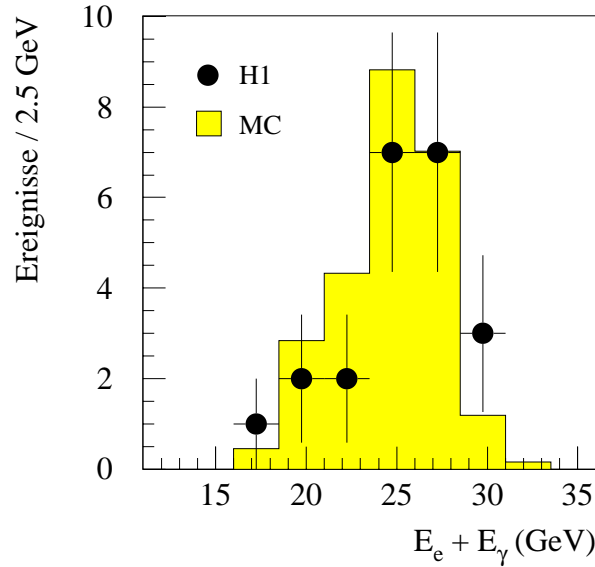
Abb. 4.13: Summenspektrum gebildet aus Elektron- und Photonenergie Die Verteilung der gemessenen Ereignisse hat die gleiche Form wie die Monte-Carlo-Verteilung (MRSD-), die auf die Anzahl der selektierten Ereignisse normiert wurde.
