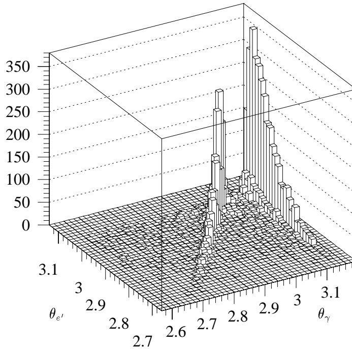
Abb. 2.4: Die Winkelverteilung von abgestrahlten Photonen
