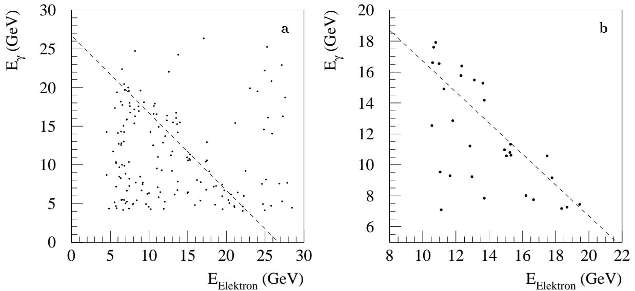
Abb. 4.2: Korrelation von Photon- und Elektronenergie bei radiativen Ereignis-Kandidaten
