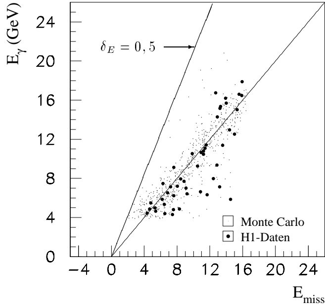
Abb. 4.6: Untergrundunterdrückung mit Hilfe von E_{ET} und E_{miss}
