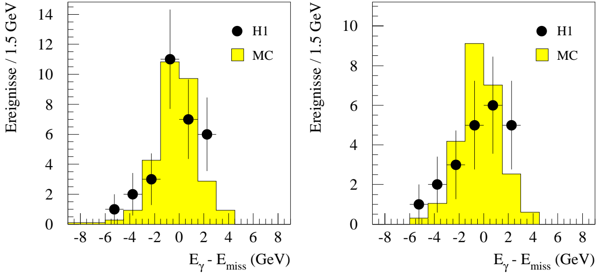
Abb. 4.8: E_{miss} -Verteilung bei radiativen Ereignissen
