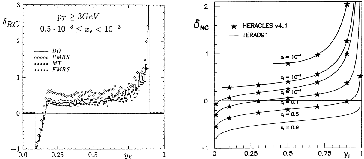
Abb. 2.6: Leptonische Korrekturen zum Wirkungsquerschnitt
