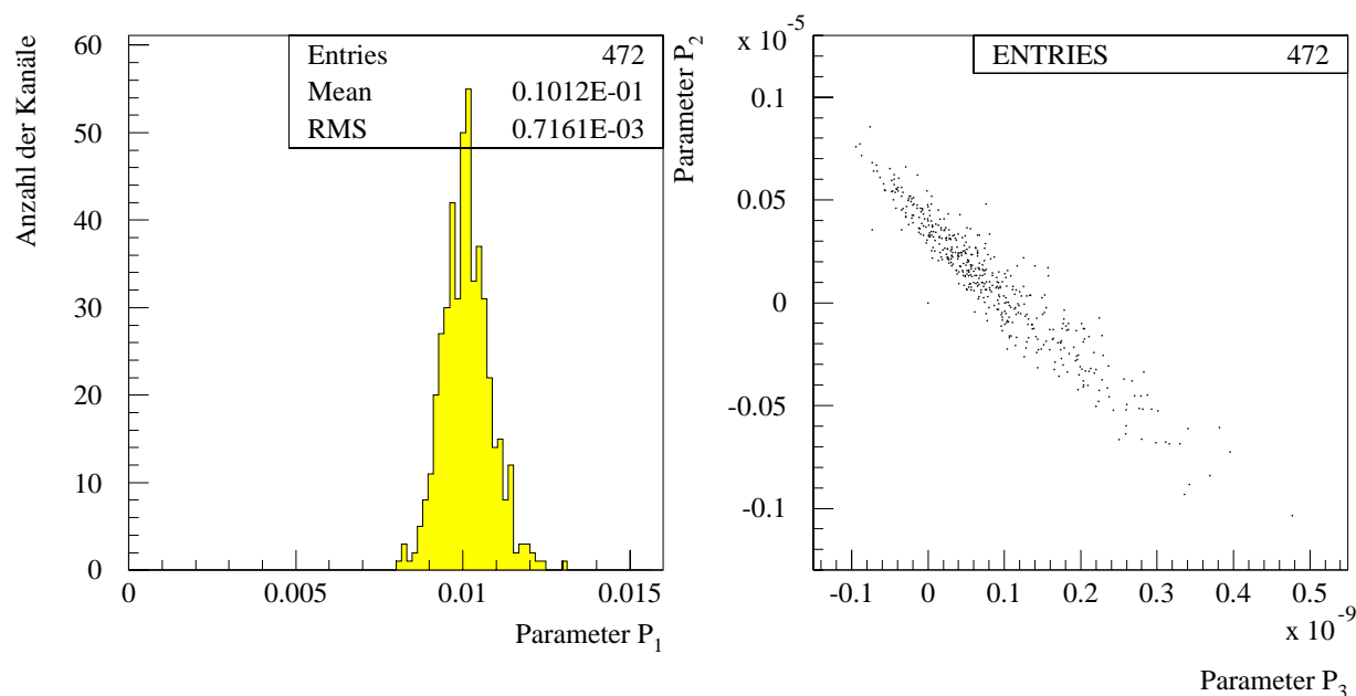
Abb. A.7: Kalibrationsparameter bei Korrektur 3. Ordnung
