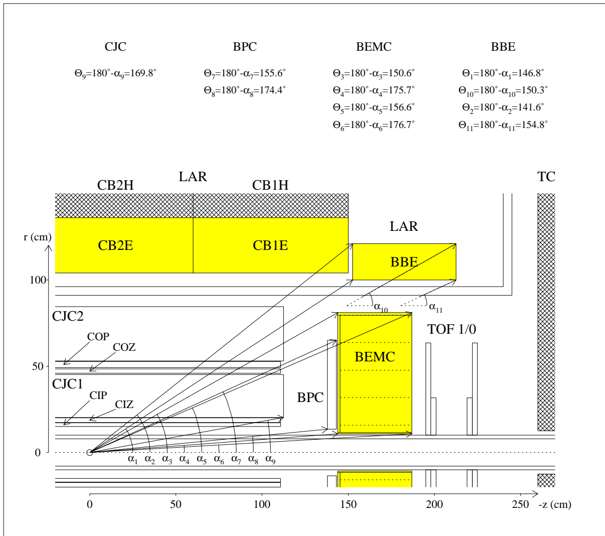
Abb. 3.11: Der Rückwärtsbereich des H1-Detektors
