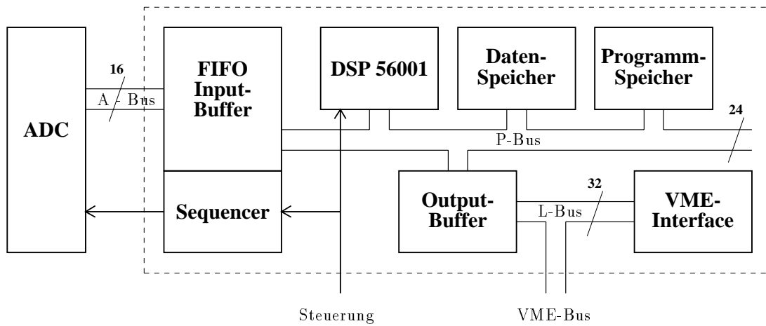
Abb. A.12: Die Architektur der in H1 benutzten DSP-Steckkarte
