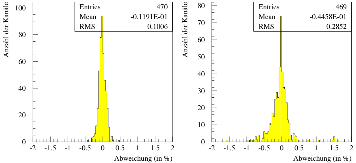
Abb. A.10: Stabilität der Elektronik bei 1500 ADC-Einheiten links: Kurzzeit-Stabilität; rechts: Langzeit-Stabilität.
