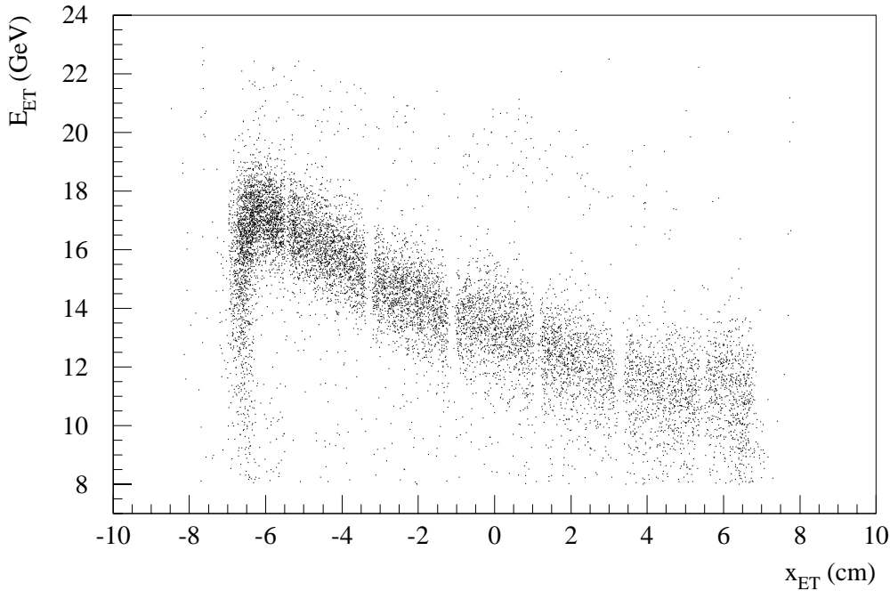
Abb. 3.9: Akzeptanz des Elektron-Taggers
