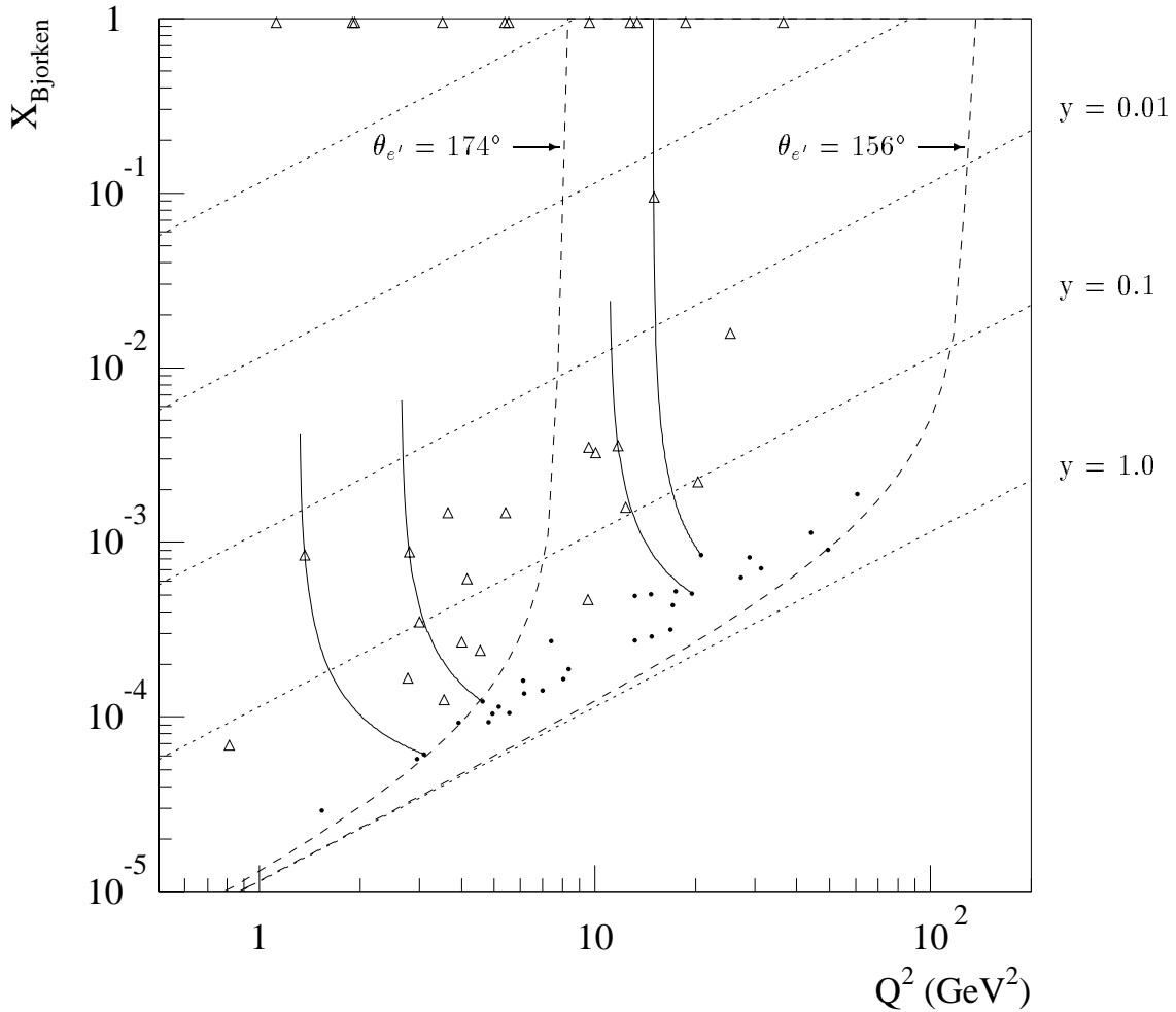
Abb. 4.12: Migration in der kinematischen Ebene durch kollineare ISR
