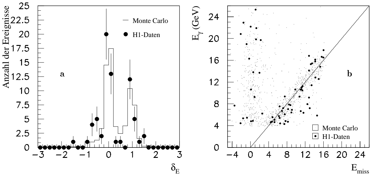
Abb. 4.4: Verteilungen ohne Untergrundunterdrückung
