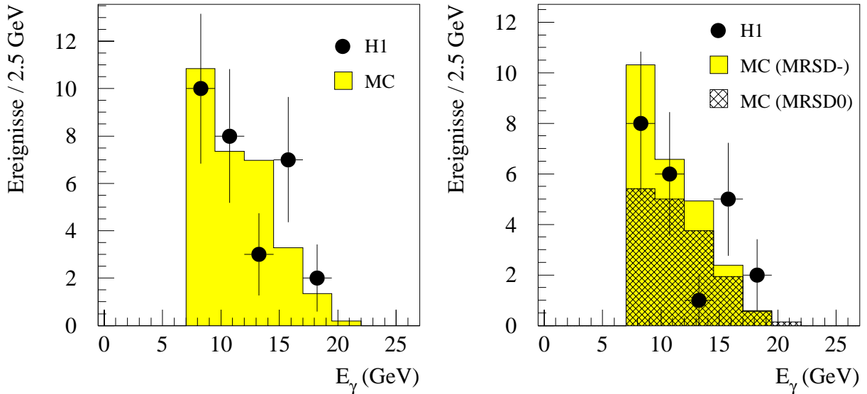
Abb. 4.10: Energiespektren von Photonen bei kollinearer ISR
