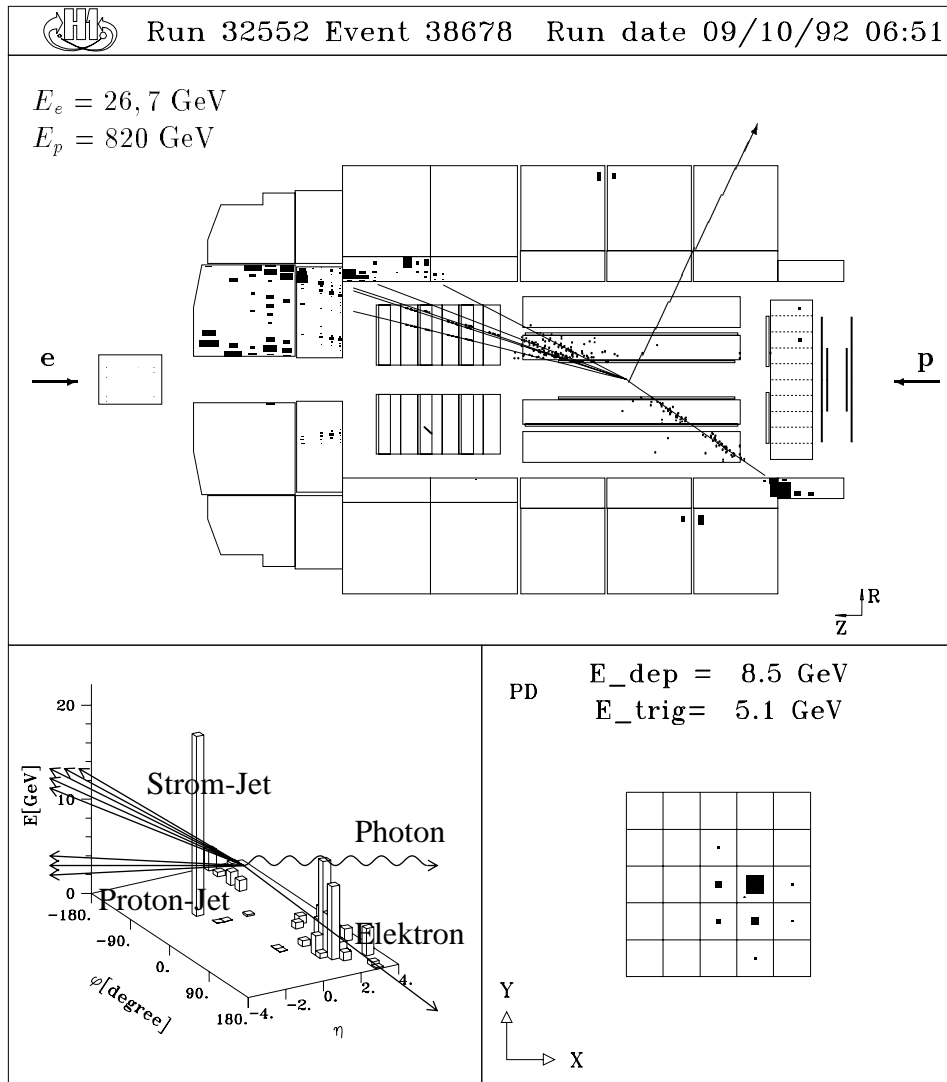
Abb. 1.3: Tief inelastisches Ereignis mit Abstrahlung eines Photons
