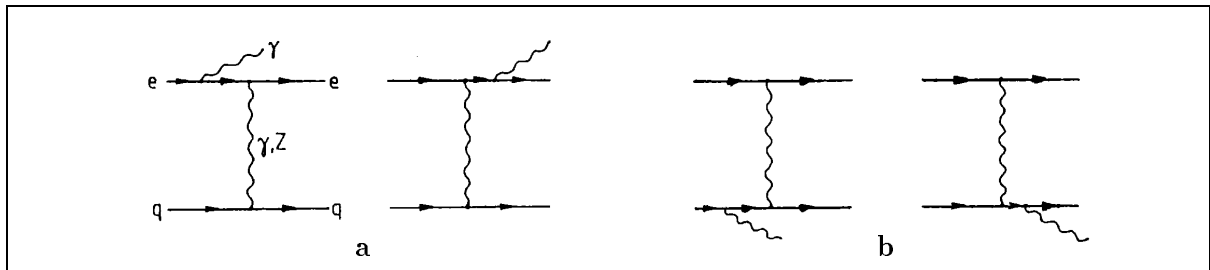
Abb. 2.2: Diagramme für die Ein-Photon-Bremsstrahlung
