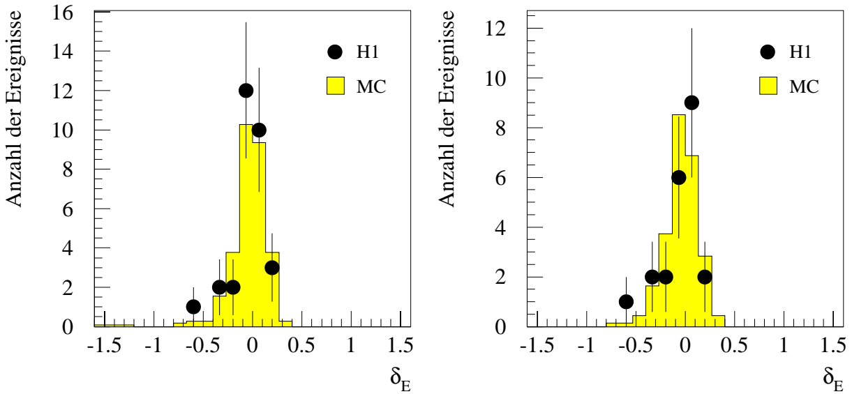
Abb. 4.9: \delta_E -Verteilung bei radiativen Ereignissen
