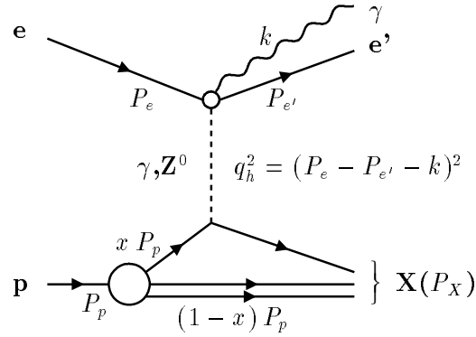
Abb. 2.5: Diagramm der harten Bremsstrahlung bei Bremsstrahlung des ein- oder auslaufenden Elektrons
