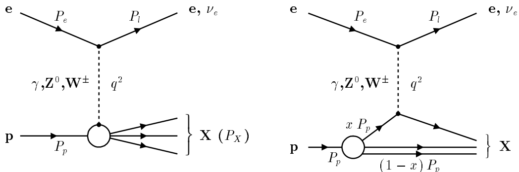
Abb. 2.1: Die tief inelastische ep-Streuung in niedrigster Ordnung links dargestellt ohne Annahme über die Struktur des Protons, rechts dargestellt entsprechend dem Quark-Parton-Modell.
