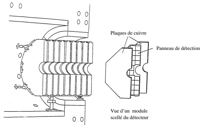
FIG. 2.17 – Bouchon calorimétrique de H1 (PLUG).
