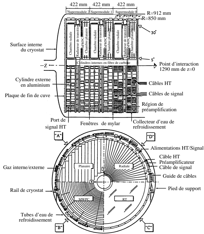
FIG. 2.8 – Schéma d'un détecteur de traces avant (FTD).
