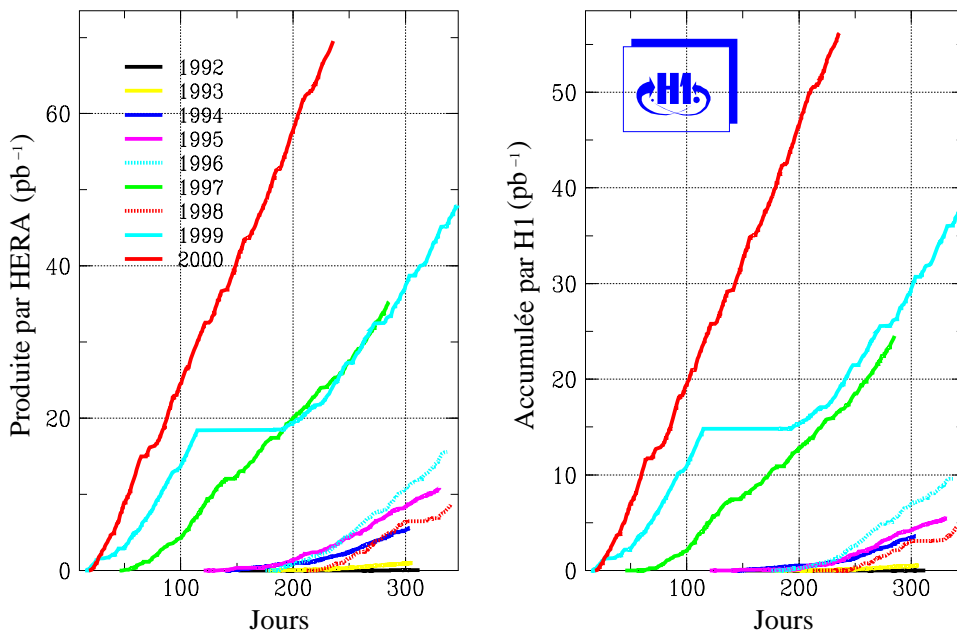
FIG. 2.2 – Luminosité accumulée produite par HERA (à gauche) et enregistrée par H1 (à droite), pour chaque année de prise de données.
