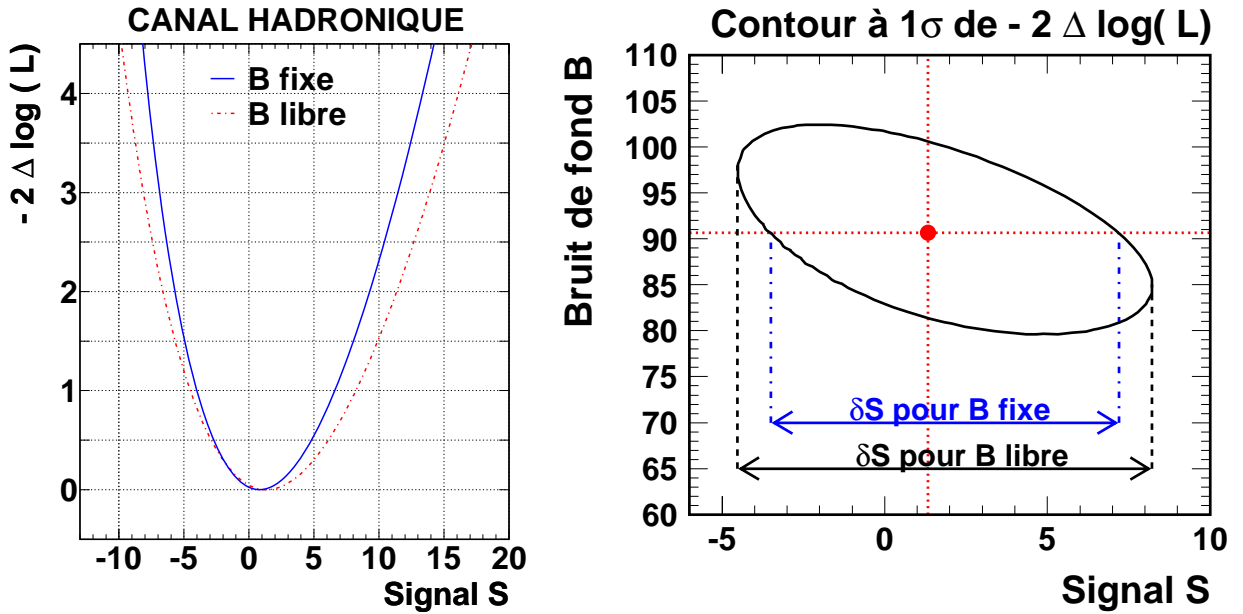
FIG. 5.15 – Ajustement -2\Delta \log \mathcal{L} en fonction de la normalisation du signal S , pour le canal hadronique, en conservant la normalisation au bruit B fixe et en variant B (figure de gauche). Contour bi-dimensionnel de la fonction -2\Delta \log \mathcal{L} à 1\sigma en fonction des normalisations au signal et au bruit S et B (figure de droite).
