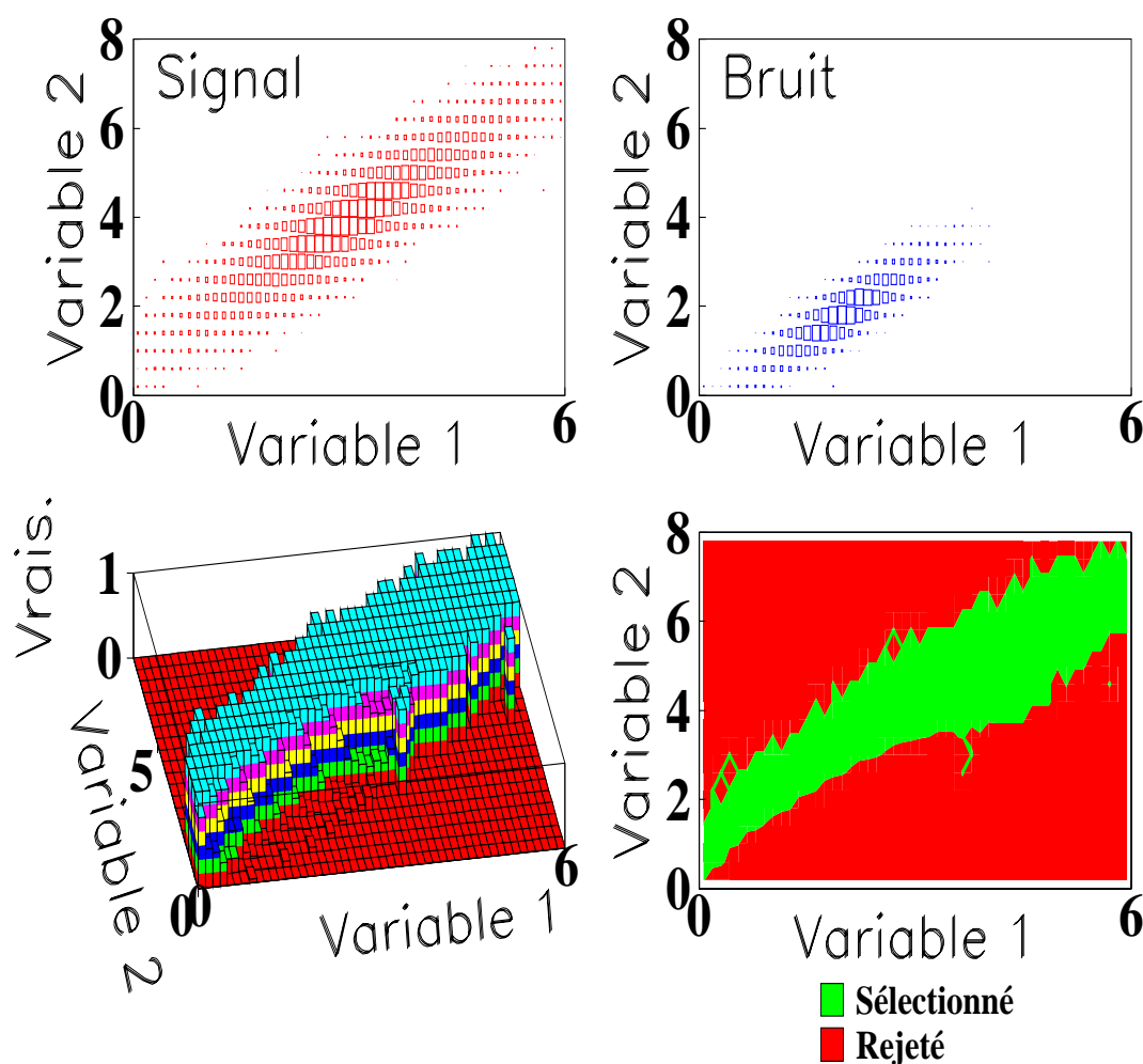
FIG. B.11 – Distribution bi-dimensionnelle des variables d'entrée de la fonction de vraisemblance pour le signal et pour le bruit (figures du haut) ; vraisemblance en fonction des variables d'entrée (figure du bas à gauche) ; vraisemblance coupée à 0.8 sur la vraisemblance en fonction des variables d'entrée (figure du bas à droite).
