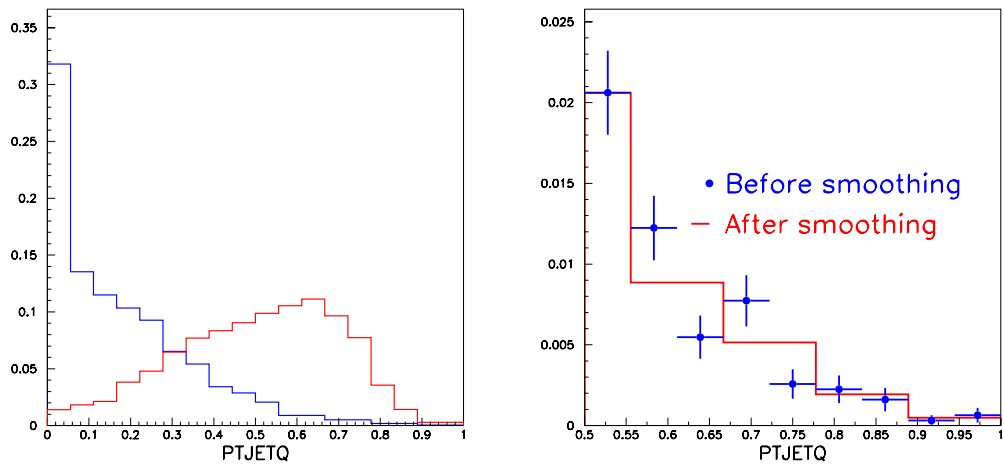
FIG. B.10 – Effet de l'association de deux intervalles de plus de 15% d'erreur sur les distributions de la variable d'entrée et de la vraisemblance résultante.
