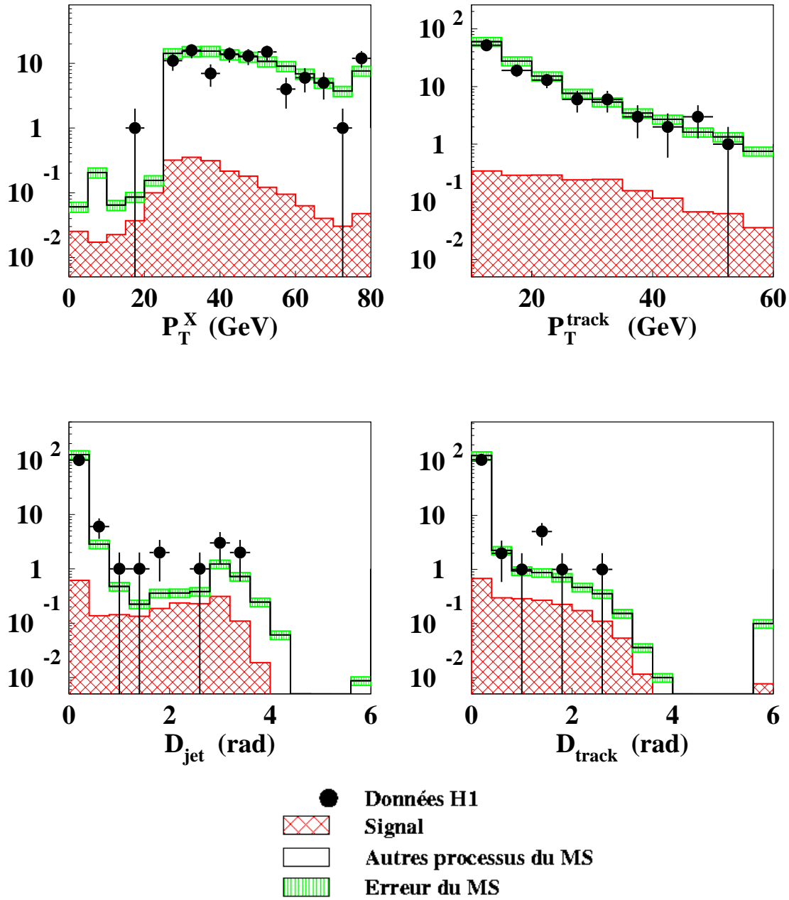
FIG. 4.22 – Distributions de l'impulsion transverse hadronique P_T^X , de l'impulsion transverse de la trace candidate P_T^{track} et de son isolation par rapport aux jets et aux traces, D_{jet} et D_{track} , pour l'échantillon de fuite de jets (données e^+p , 104.7 \text{ pb}^{-1} ). Le dernier intervalle des distributions en P_T^X , D_{jet} et D_{track} contient tous les événements dont les valeurs de P_T^X , D_{jet} et D_{track} est au-dessus de la limite supérieure de l'histogramme.
