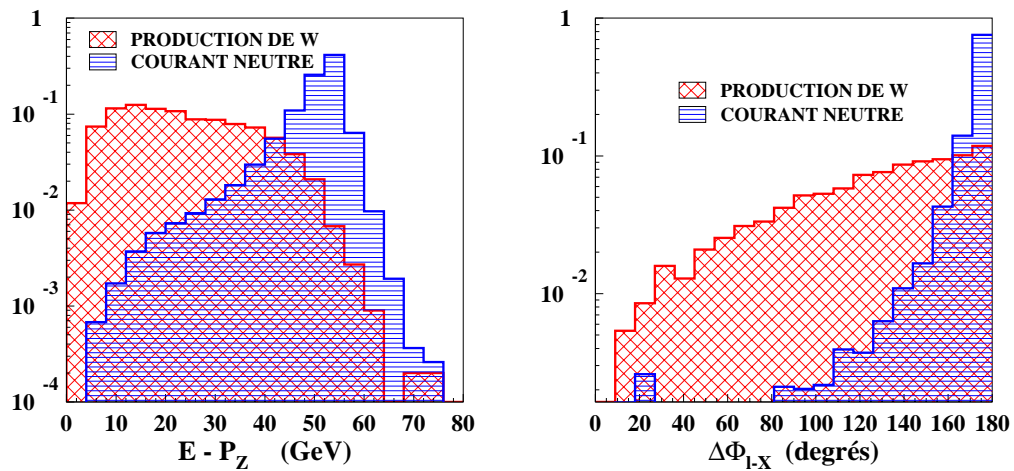
FIG. 4.5 – Distribution de E - P_z (figure de gauche) et de l'acoplanarité \Delta\Phi_{\ell-X} (figure de droite) pour la production de W \rightarrow e\nu et le bruit de fond à courant neutre (échelle verticale arbitraire).
