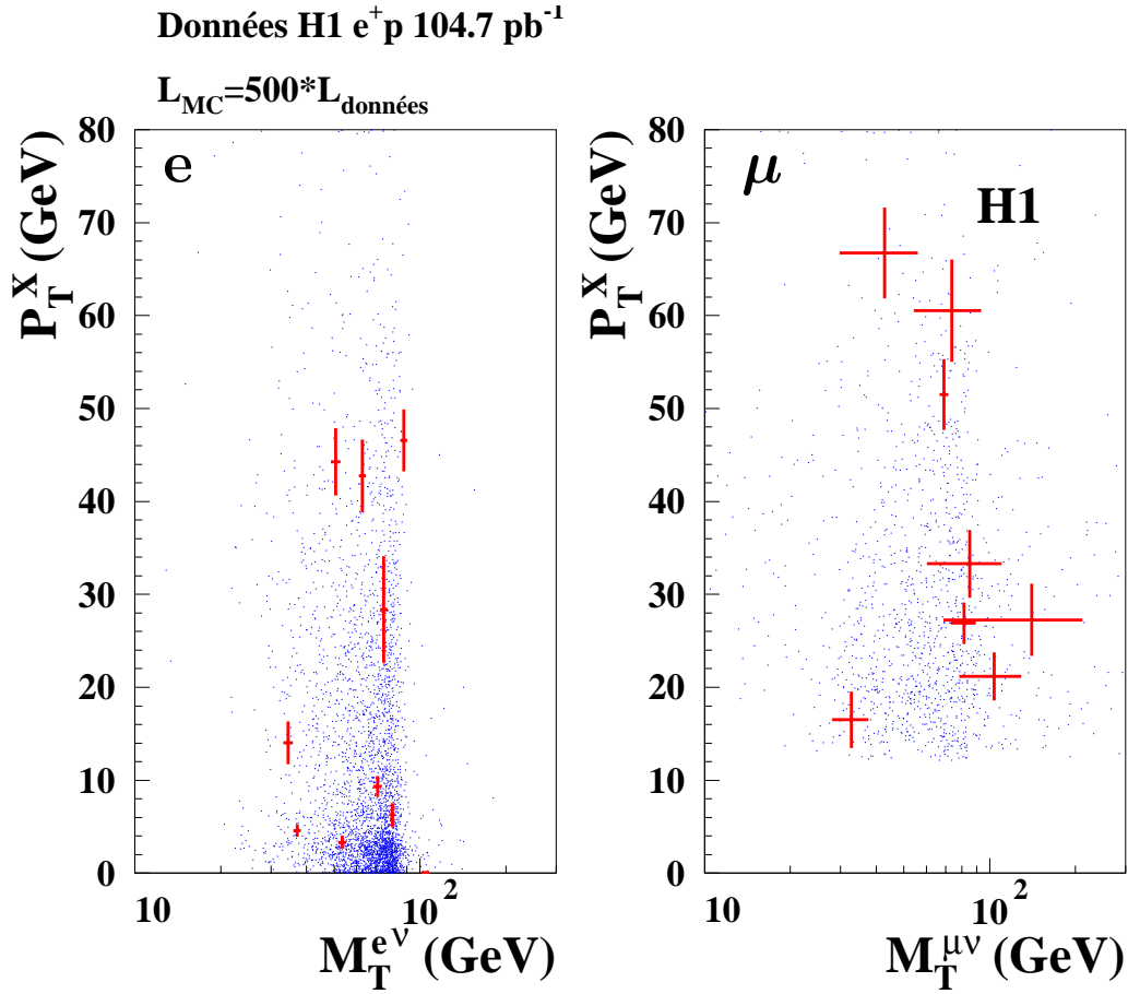
FIG. 4.16 – Distribution de l'impulsion transverse du système hadronique des événements en fonction de la masse transverse M_T^{lν} , pour le canal électron (figure de gauche) et le canal muon (figure de droite). Les croix représentent les candidats sélectionnés avec leurs erreurs et les points correspondent à la prédiction du signal simulée pour une luminosité de 500 fois la luminosité des données.
