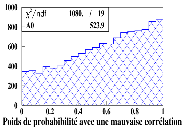
FIG. B.4 – Distribution du poids de probabilité des fonctions tests simulant le signal avec une bonne reconstruction de la corrélation (0.9) entre les variables d'entrée (figure du haut) et une mauvaise reconstruction de cette corrélation artificiellement posée à 0.7 (figure du bas).
