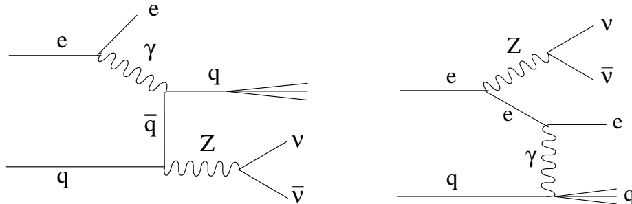
FIG. 3.11 – Diagrammes de production du boson Z dans les collisions ep avec désintégration en deux neutrinos.
