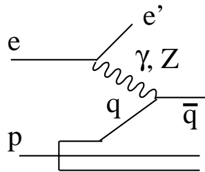
FIG. 3.12 – Diffusion profondément inélastique à courant neutre.
