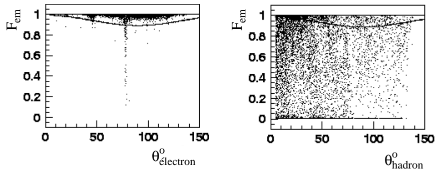
FIG. 2.11 – Spectre de la fraction électromagnétique F_{EM} en fonction de l'angle polaire de l'amas, pour des amas d'électrons (figure de gauche) et des amas de hadrons (figure de droite). La courbe continue représente la coupure F_{EM}^{min} au-dessus de laquelle les amas sont sélectionnés.
