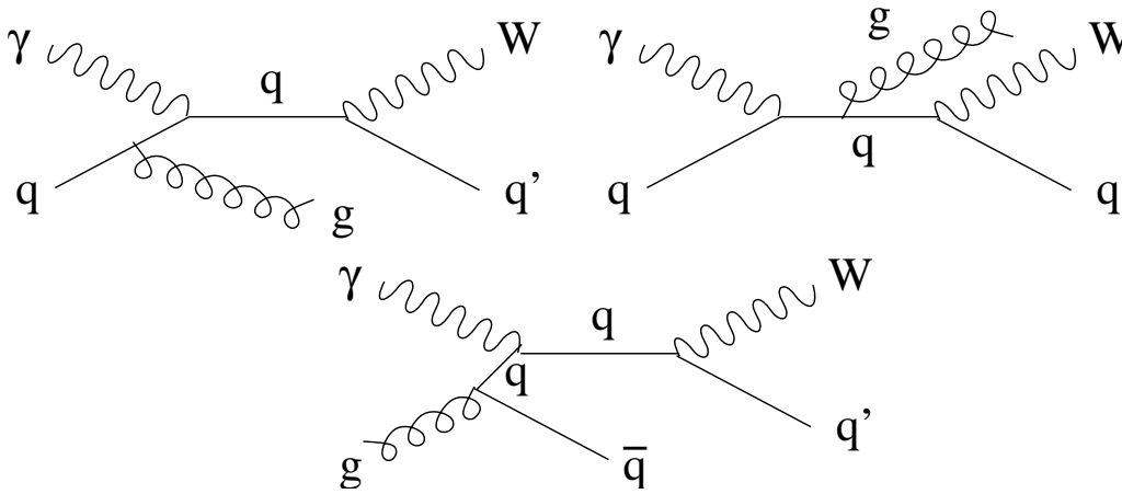
FIG. 3.8 – Diagrammes typiques de corrections réelles sur la production de W .
