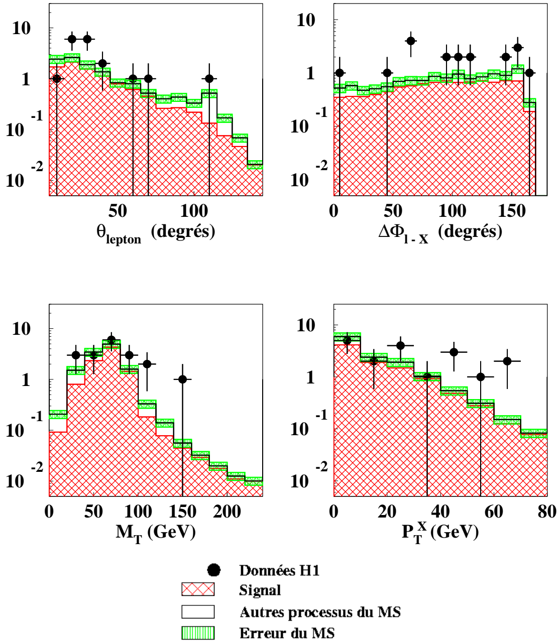
FIG. 4.12 – Distribution de l'angle polaire du lepton \theta_{\text{lep}} , de l'acoplanarité \Delta\Phi_{\ell-X} , de la masse transverse M_T^{\ell\nu} du système lepton-neutrino et de l'impulsion transverse hadronique P_T^X pour les canaux électron et muon combinés (données e^+p , 104.7 \text{ pb}^{-1} ).
