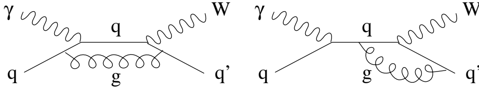
FIG. 3.7 – Diagrammes typiques de corrections virtuelles sur la production de W .
