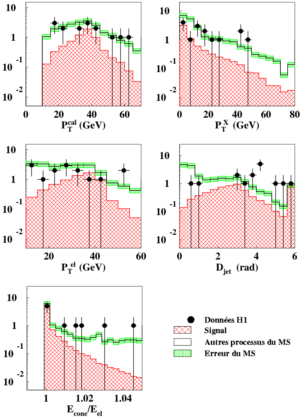
FIG. 4.18 – Distributions de contrôle dans le canal électron pour l'échantillon enrichi en courants chargés (données e^+p , 104.7 \text{ pb}^{-1} ). Le dernier intervalle de la distribution en P_T^X ( D_{jet} ) contient tous les événements dont la valeur de P_T^X ( D_{jet} ) est au-dessus de la limite supérieure de l'histogramme.
