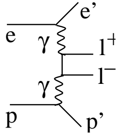
FIG. 3.16 – Production de paires de leptons.
