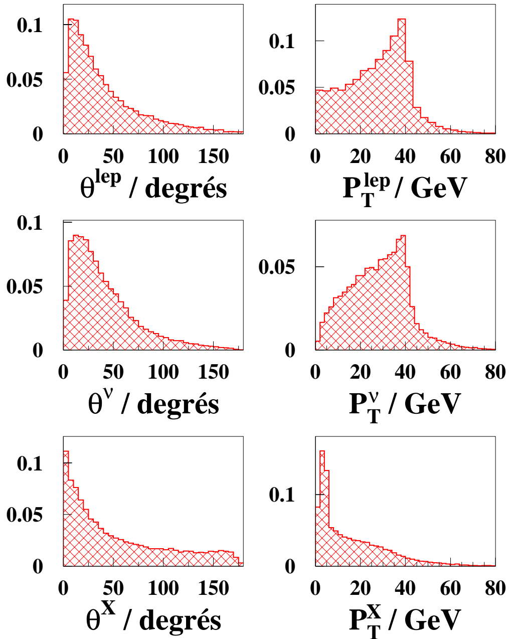
FIG. 3.4 – Distributions de l'angle polaire (colonne de gauche) et de l'impulsion transverse (colonne de droite) du lepton, du neutrino et du jet issus du boson W, simulés par le générateur EPVEC pour le processus e^\pm p \rightarrow eW^\pm + X (échelle verticale arbitraire).
