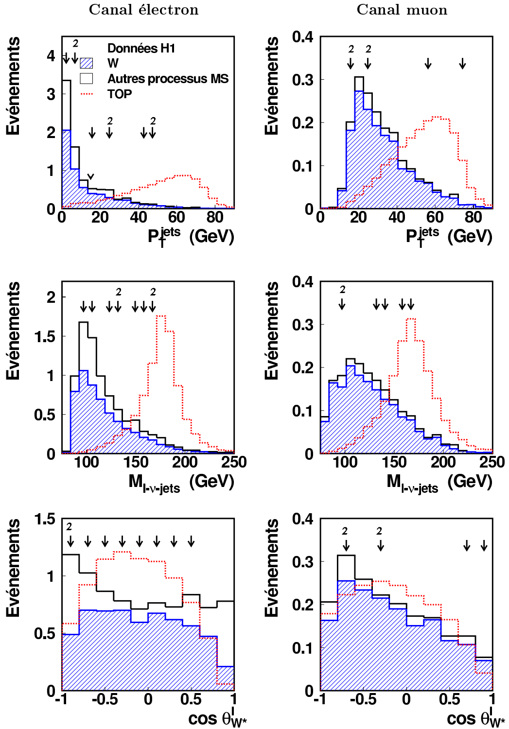
FIG. 5.6 – Pour chacun des deux canaux, distributions de la somme de l'impulsion transverse des jets P_T^{\text{jets}} , de la masse du système lepton-neutrino-jet M_{\ell-\nu\text{-jets}} et du cosinus de l'angle de désintégration du W dans son centre de masse \cos \theta_{W^*}^{\ell} pour la production de top (histogrammes pointillés), le Modèle Standard (histogrammes pleins) et les données expérimentales (flèches; les chiffres au-dessus des flèches indiquent le nombre d'événements de données dans l'intervalle concerné). Ces distributions sont effectuées après la présélection top, pour l'ensemble des données de HERA-1 ( 118.3 \text{ pb}^{-1} ).
