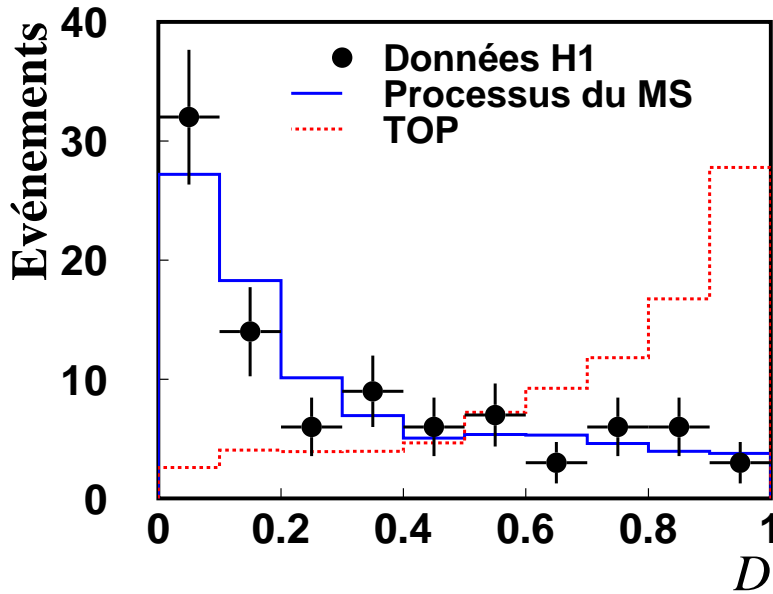
FIG. 5.13 – Distribution de la vraisemblance obtenue dans le canal hadronique, obtenue à partir des variables d'entrée P_T^{jets} , \cos \theta_W^* et M_{jets} , sur l'ensemble des données e^\pm p de HERA-1 ( 118.3 \text{ pb}^{-1} ).
