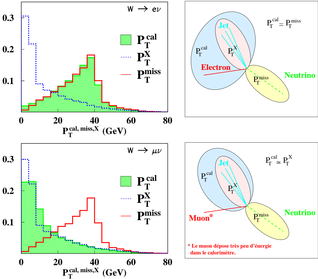
FIG. 4.4 – Figures de gauche : distributions des impulsions transverses P_T^{cal} , P_T^X et P_T^{miss} pour la prédiction de production de W pour les canaux électron ( W \rightarrow e\nu ) et muon ( W \rightarrow \mu\nu ) (échelle verticale arbitraire). Figure de droite : Vue transverse des objets considérés dans le calcul de chacune de ces variables, pour chacun des deux canaux (ces figures supposent que l'électron diffusé n'est pas détecté).
